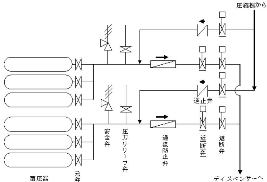
図 1. 蓄圧器配管集合部の例
