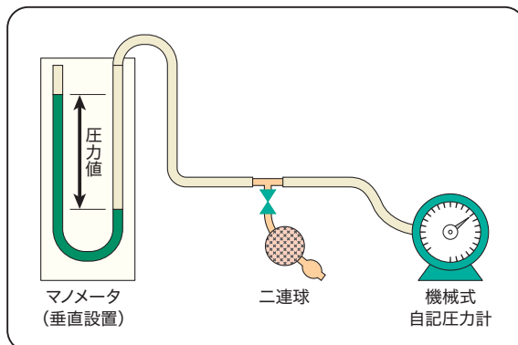
水柱マンメータ検査方法
