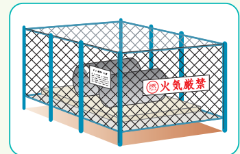
図3-3 さく設置例
