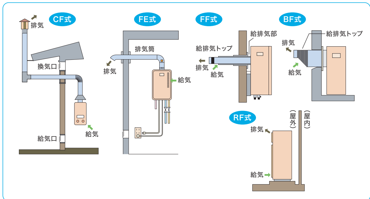
図4-12 給排気形式による分類
