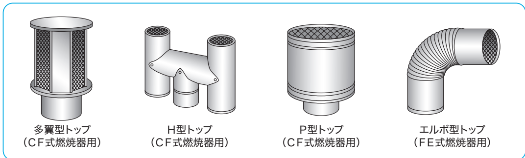
図4-15 排気トップの例
