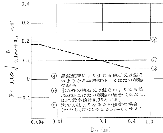
Rf と粒径の関係図
