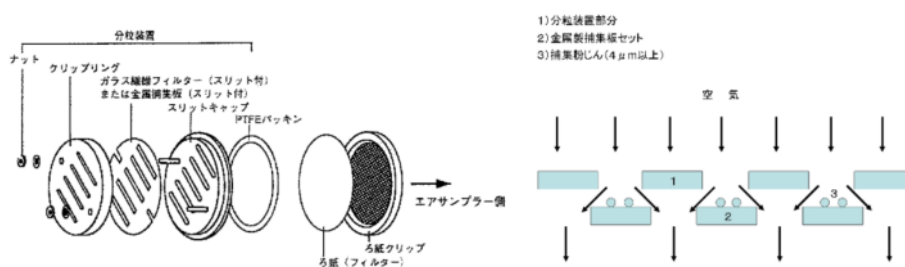
図 22 HV-500F 型の慣性衝突式
