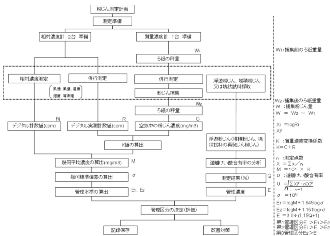
図2 粉じん濃度測定のフローチャート
