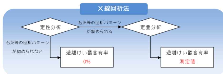
図 11 X線回析法の流れ
