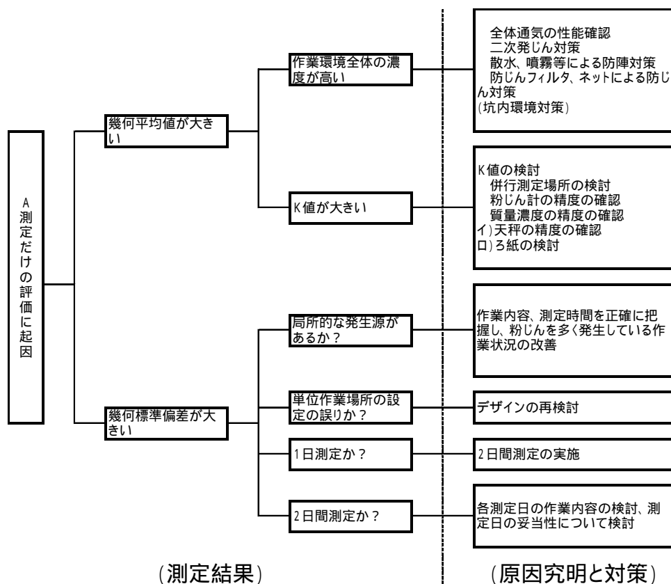
図 16 原因究明と改善対策フローシート
