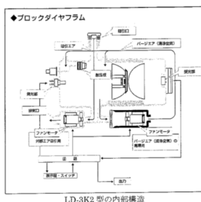
図 24 構造図
