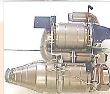
排気後処理システム “DPF with SCR Assy”
