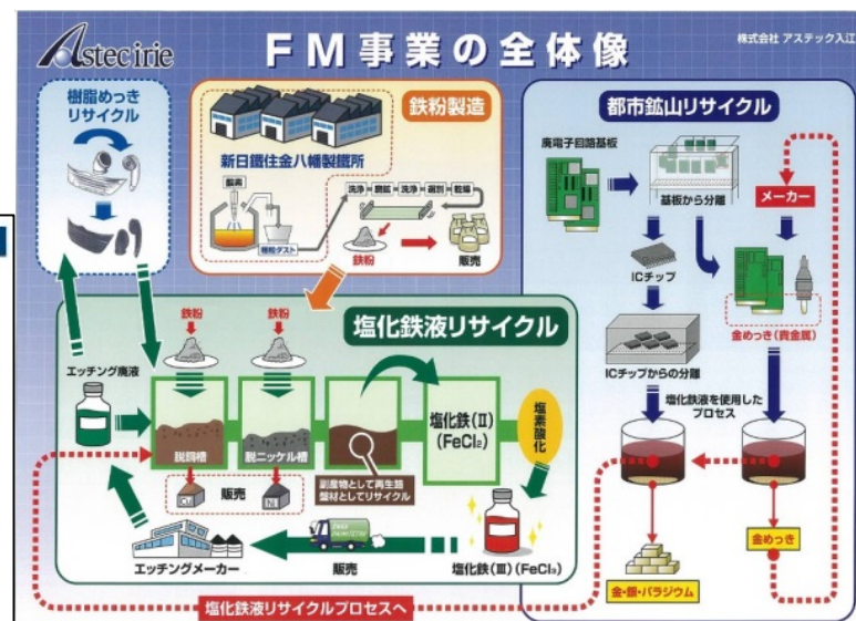
独自の塩化鉄・都市鉱山リサイクルのフロー
