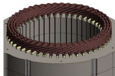
新型モーター（平角線コイル）
