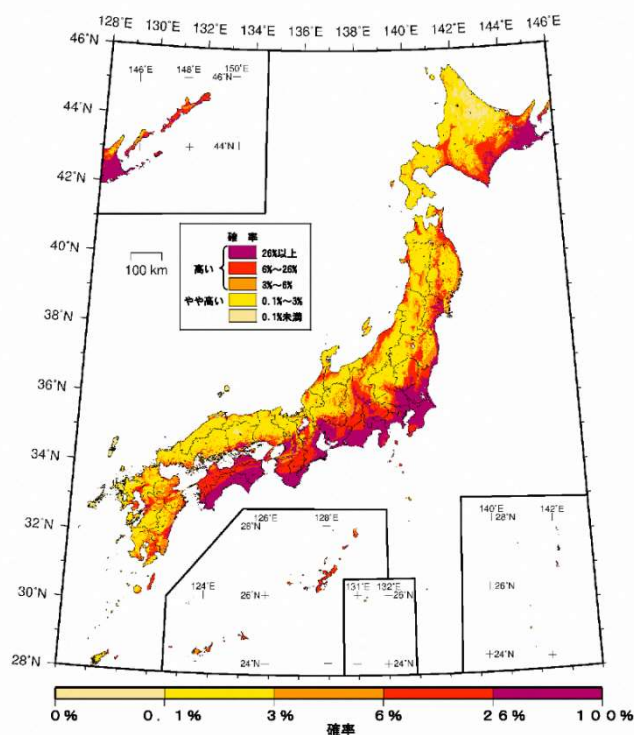
今後30年間に震度6弱以上の揺れに見舞われる確率（平均ケース・全地震）
