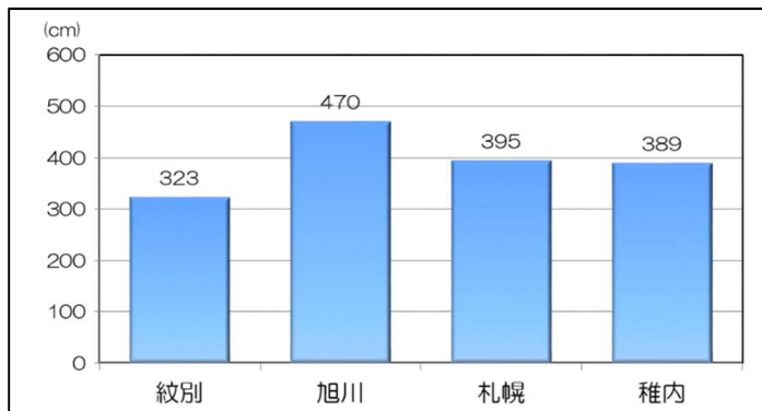
平成30年から令和4年の年間総降雪量（平均値）
