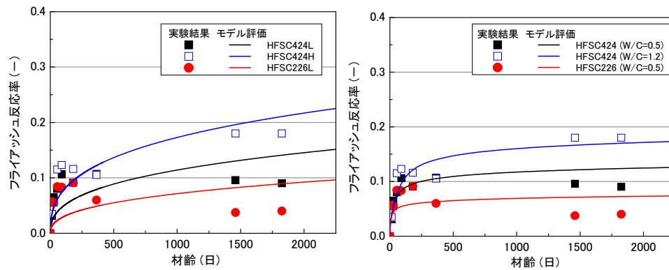
(図3-100) Shrinking Coreモデルによるフライアッシュ反応率の評価結果 (左図：既存の Shrinking Core モデル、右図：改良後の Shrinking Core モデルでの評価)
