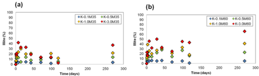
(図 3-101) スメクタイトのイライト化率の経時変化 (a) 反応温度 35°C、(b) 反応温度 60°C
