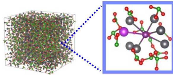
図 3-84. リバースモンテカルロ計算により得られた BPI ガラス固化体の構造モデル
