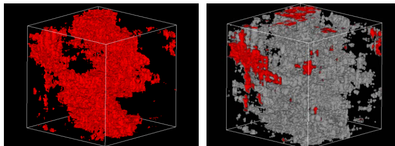
図3-68. 変質に伴う物質移行特性(拡散係数)算定手法で使用するセメント水和物と空隙構造の三次元モデル
