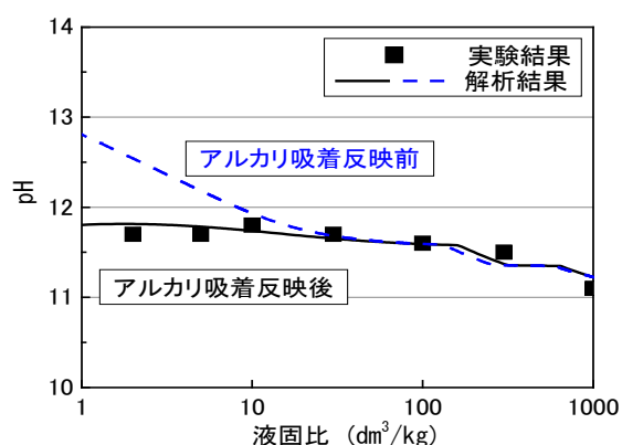
図 3-99 アルカリ吸着反映前後の水和物溶解沈殿モデルによる pH の整合性 （試製 \text{SO}_3 低含有 HFSC によるバッチ式浸漬実験の結果とその解析結果）
