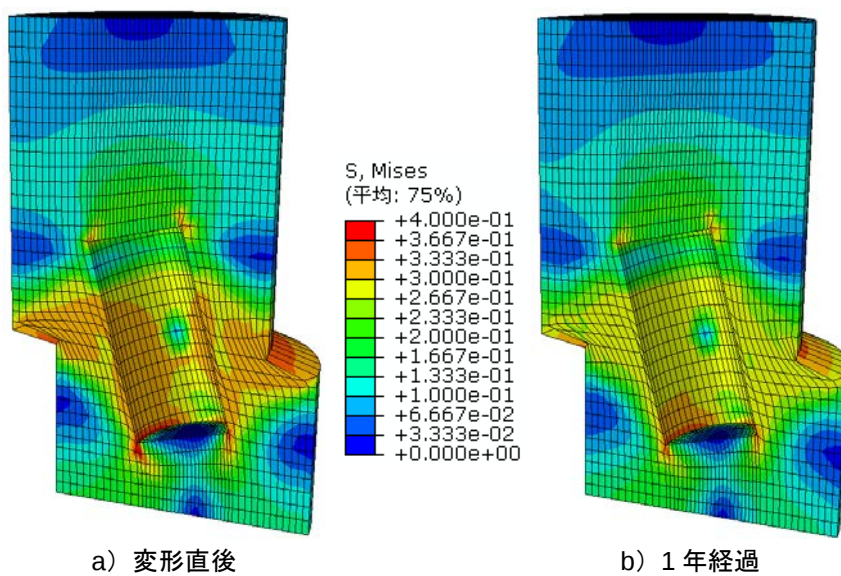
図 3 - 2 1 人工バリア限界状態試挙動（せん断）の解析例
