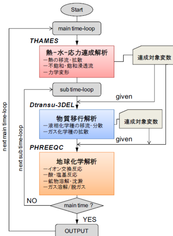
図 3-29 THMC 連成解析モデルのスキーム
