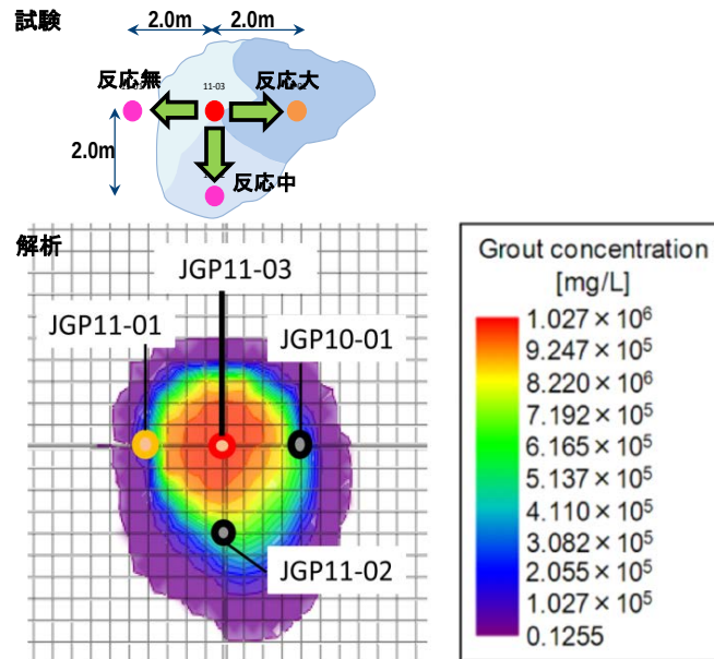
図 3-60. GTS 原位置試験に対する等価多孔質媒体モデルを用いたグラウト浸透距離の解析結果と実測値の比較
