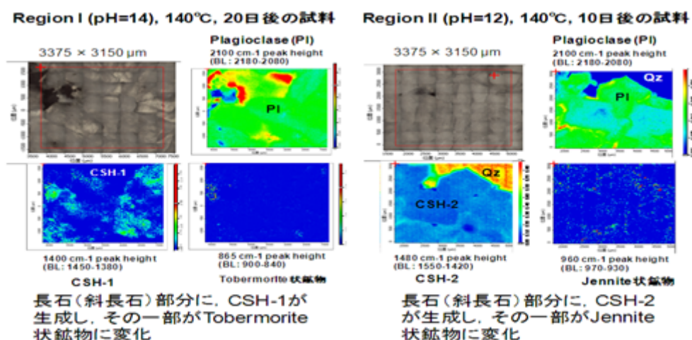
図 3－6 3. 顕微赤外分光法（面分析）による二次鉱物の分析評価の例
