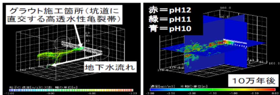
図3-6 2. セメント系グラウト材料による地下水水質への影響評価モデル解析の例
