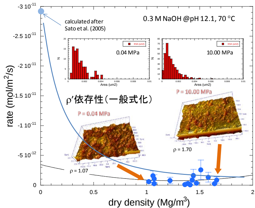
図 3-71. モンモリロナイト溶解速度と密度の関係（一般式化の一例）
