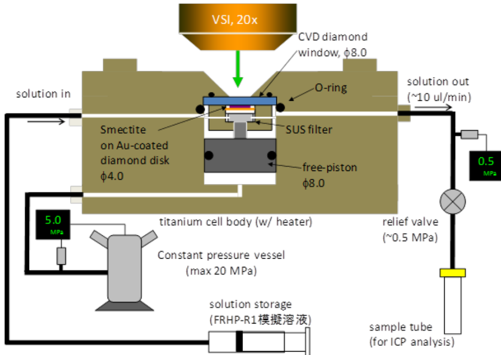
図 3-70. 自動圧縮セルとその場垂直走査干渉計計測システム
