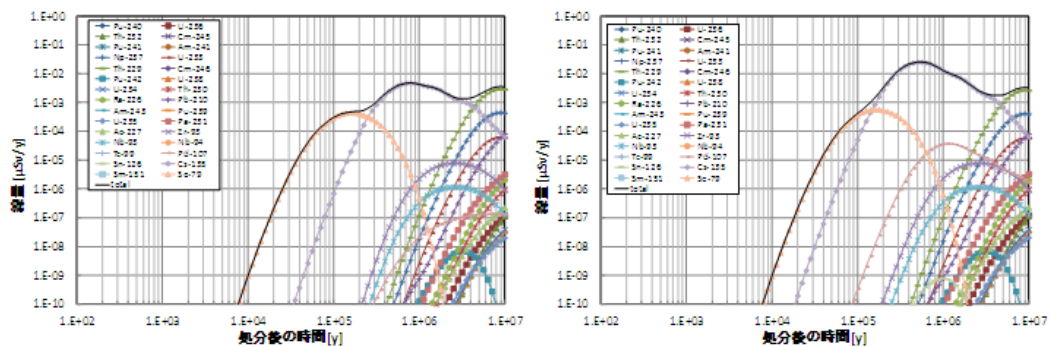
図 3-107. 硝酸塩影響評価システムによる高レベル放射性廃棄物処分の線量評価試算結果の例（左図：硝酸塩影響なし、右図：硝酸塩影響あり）
