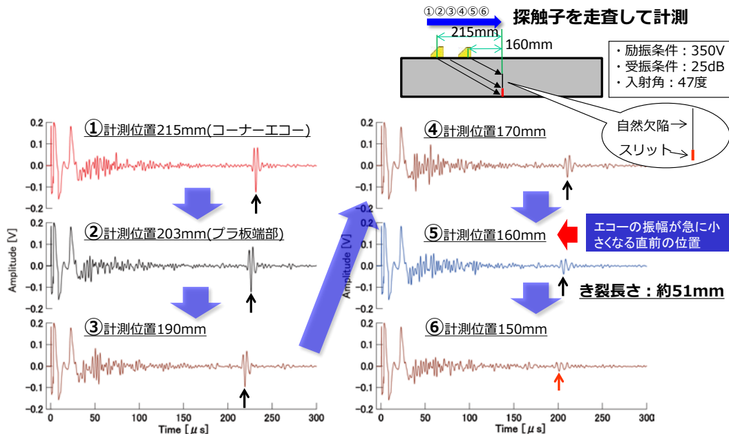
図3-89. 超音波法によるひび割れ探傷結果
