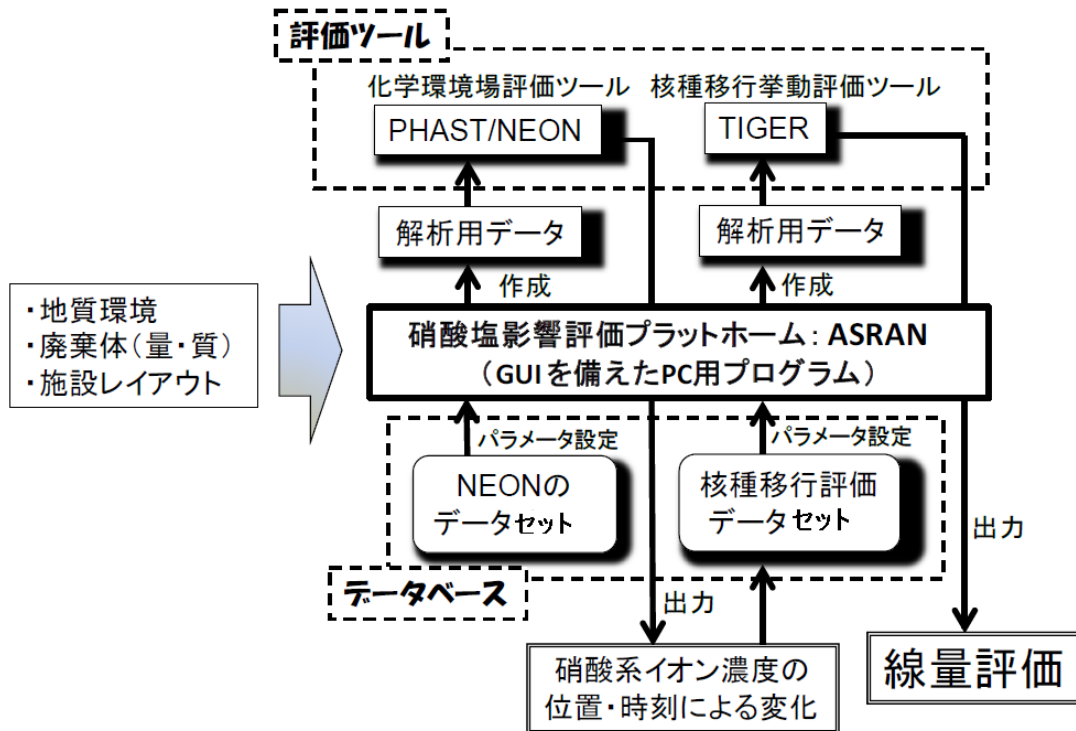
図3-106 硝酸塩影響評価システムの構成
