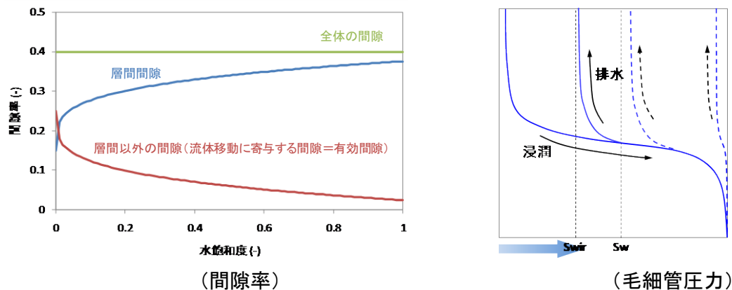
図 3-79. ベントナイトの膨潤/収縮による有効空隙率及び毛細管圧力の変化を考慮した 2 相流パラメータの概念
