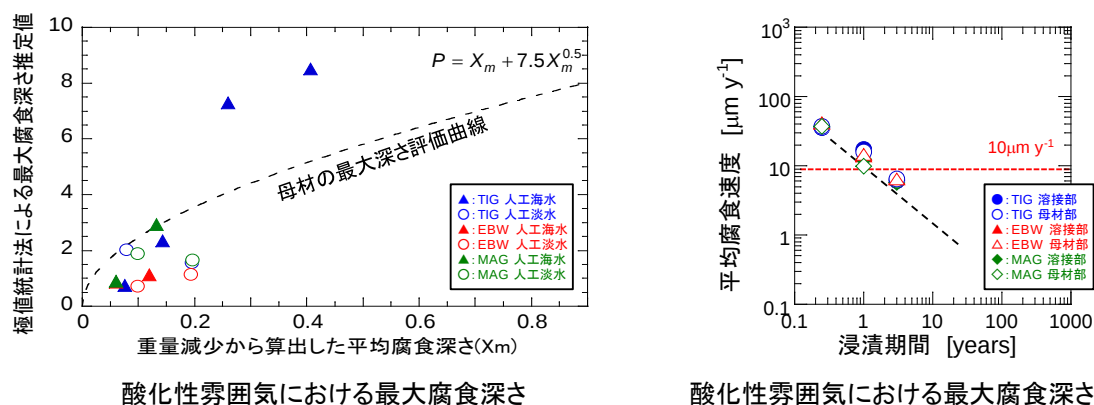
図3-42. 人工バリア品質評価・オーバーパック／ （溶接部耐食性評価試験）
