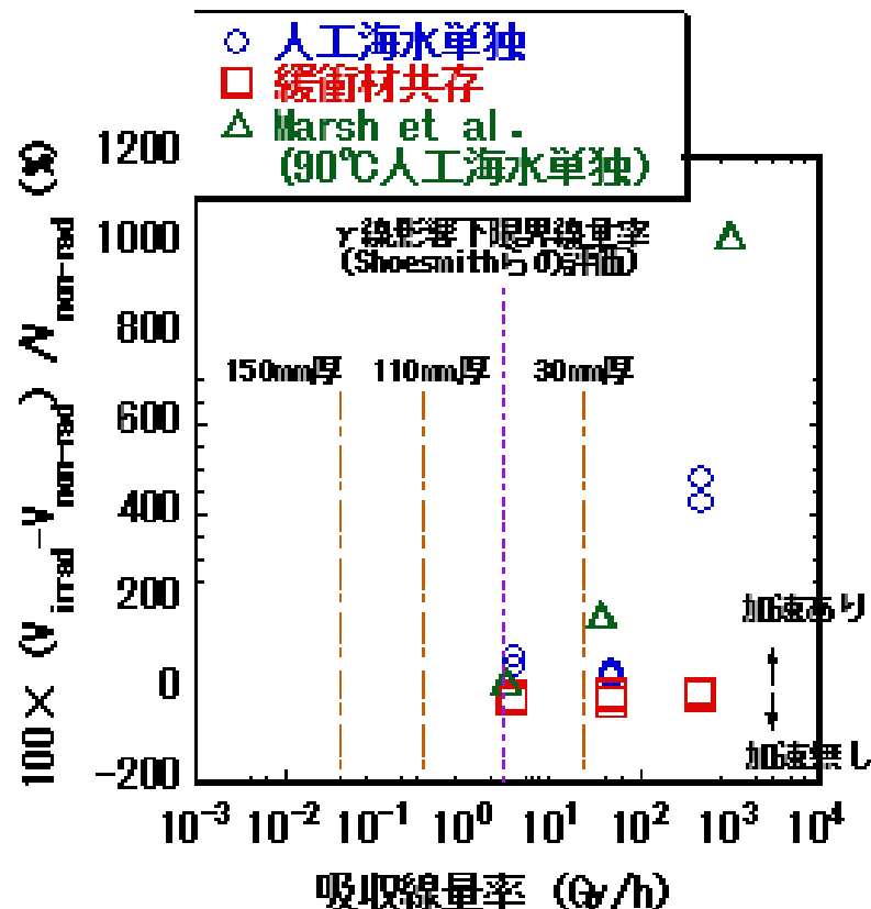
図3-2-2 吸収線量率と腐食加速度合いの関係
