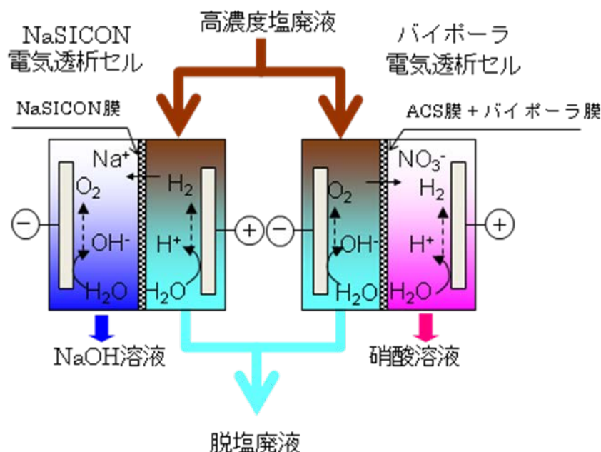
図 3 - 1 0 9 . 二電気透析セル方式の概念図
