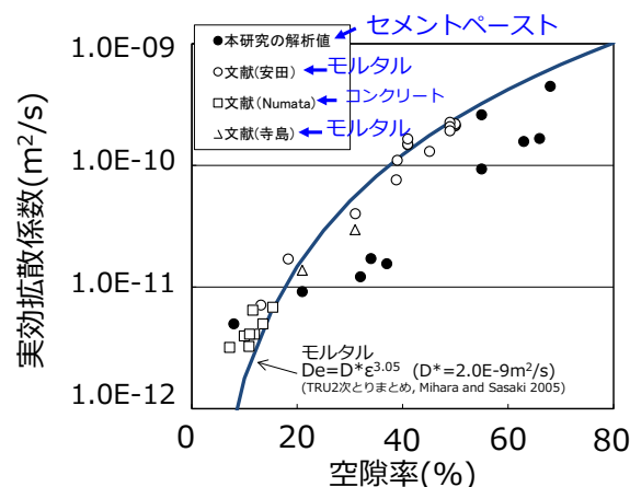
図3-69. セメント系材料の変質に伴うトリチウムの拡散係数の算出結果
