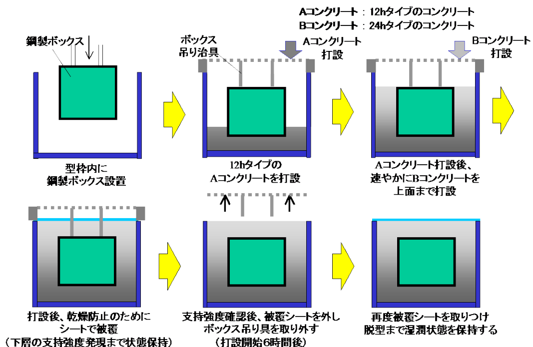
図 3-88. コンクリート容器の製作方法(一体成型法)
