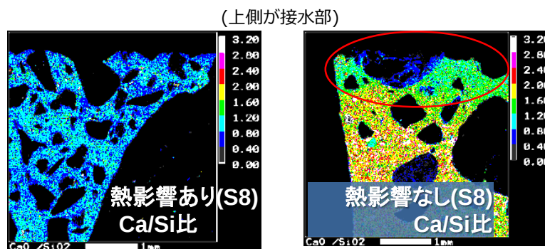
図3-66. 経年コンクリートの熱影響に伴う結晶化の進行に関するX線回折による確認結果
