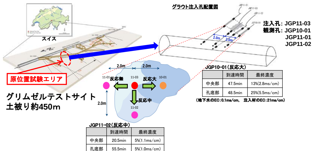
図 3-59. GTS におけるグラウト注入試験の概要と試験結果
