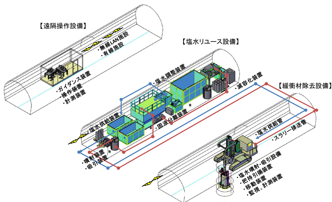
図3-51. 緩衝材除去装置の基本的な配置
