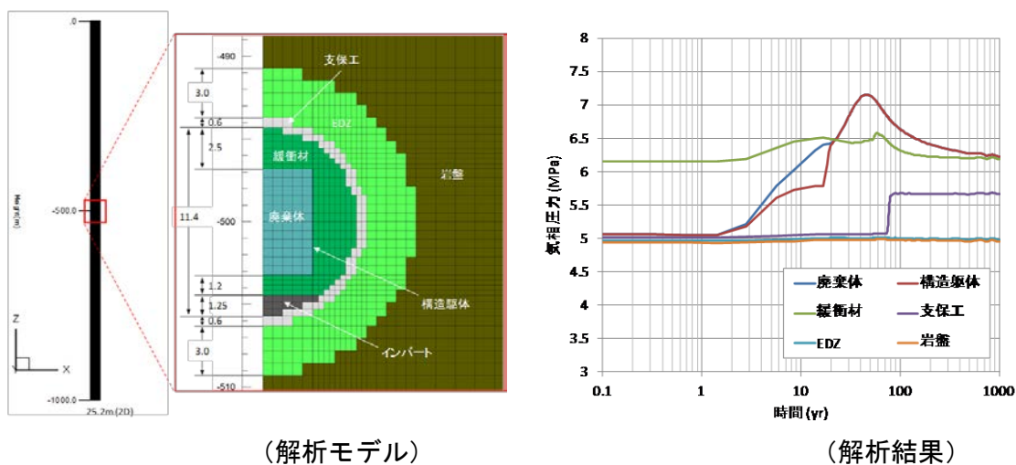
図 3-80. ガス発生を考慮した長期変遷解析における人工バリア部位毎のガス（気相）圧力の 1000 年後迄の時間変化
