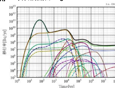
図 3-76. 人工バリアでの核種移行計算の結果
