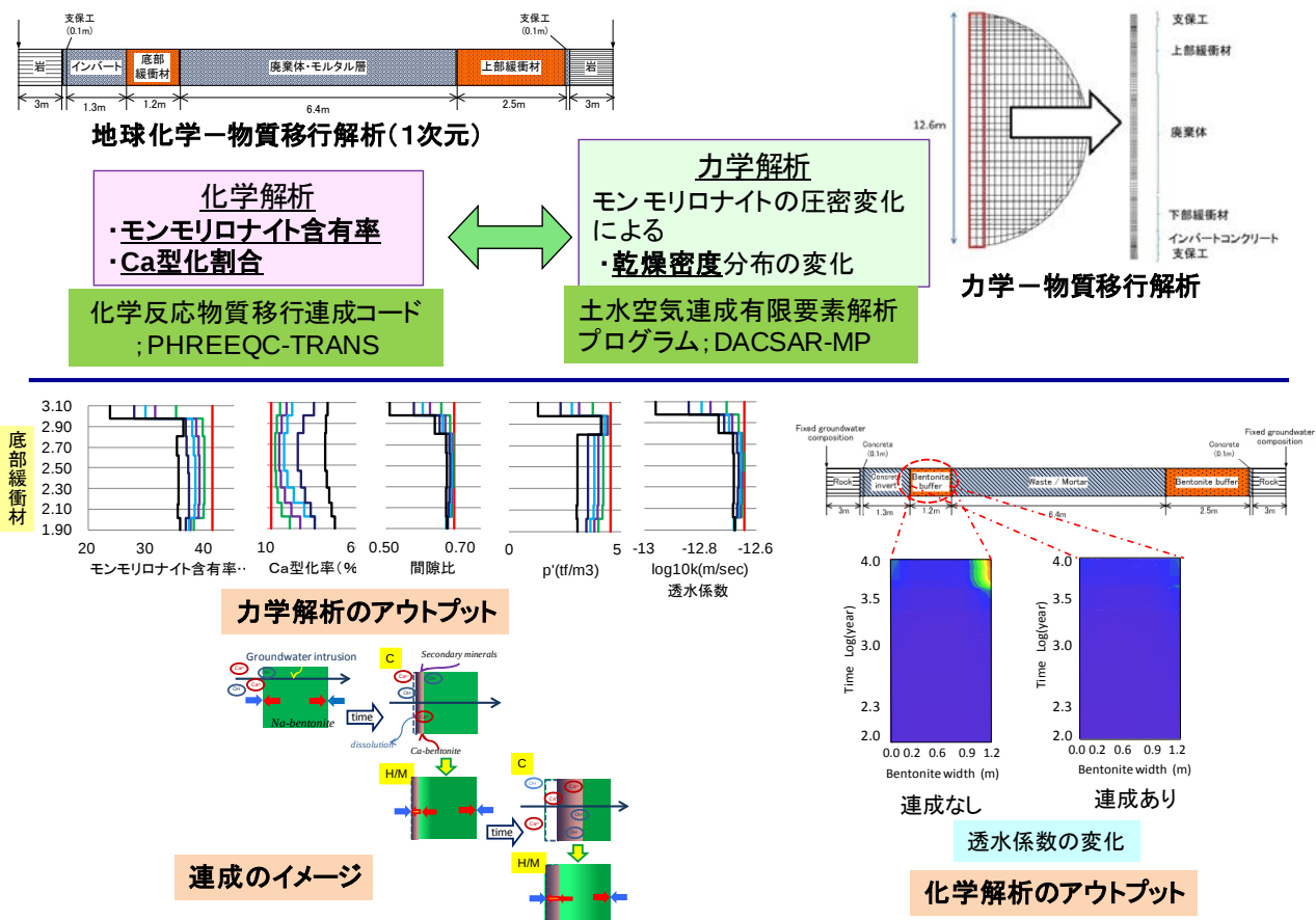
図3-75. 力学・化学連成解析の効果のまとめ
