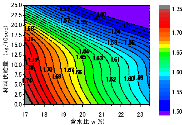
図 3-125. 吹付けベントナイトの含水比—供給量—乾燥密度の関係
