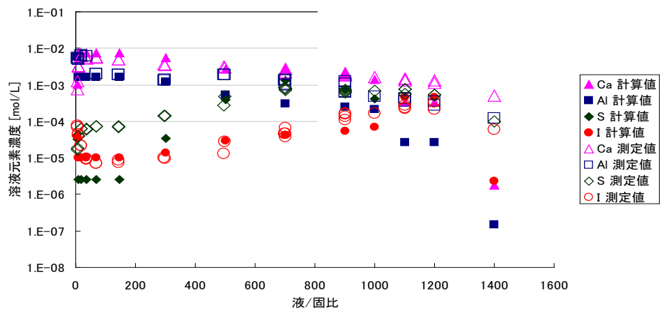
図 3－86． セメント固化体の液交換試験と、鉱物の溶解平衡に基づいたヨウ素放出モデルとの比較
