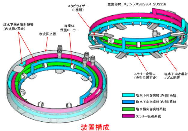
図 3 - 5 3. 塩水噴射・スラリー吸引部の構成と製作状況
