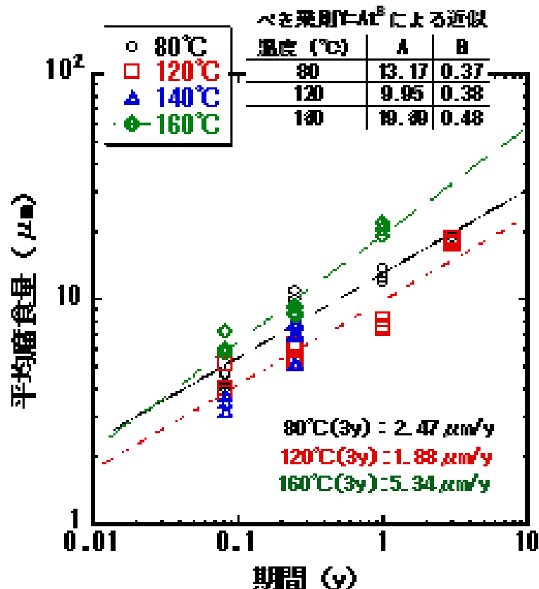
図 3-31 全面腐食挙動（還元性）試験結果 160°Cまで全面腐食（還元性）速度の顕著な増加は認められない
