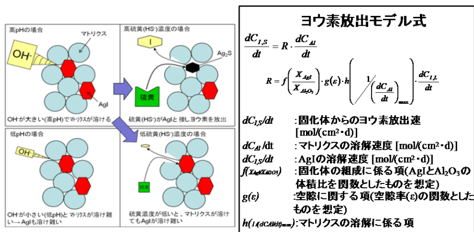
図3-83. 岩石固化体からのヨウ素放出概念（左）と評価モデル式（右）
