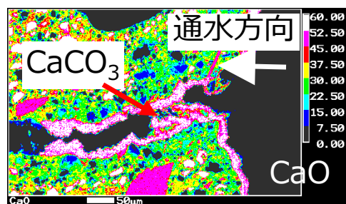
図 3－9 3. ひび割れ閉塞試験結果
