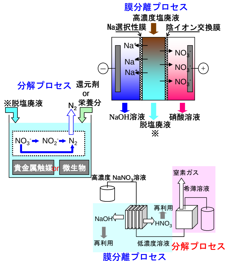
図 3-108. 放射性廃液中の高濃度硝酸塩の除去技術の概念 (膜分離プロセスで分離された硝酸ナトリウムは再処理工程で再利用される。本システムにより、再処理工程から発生する廃棄物としての硝酸塩量を削減することができる。)
