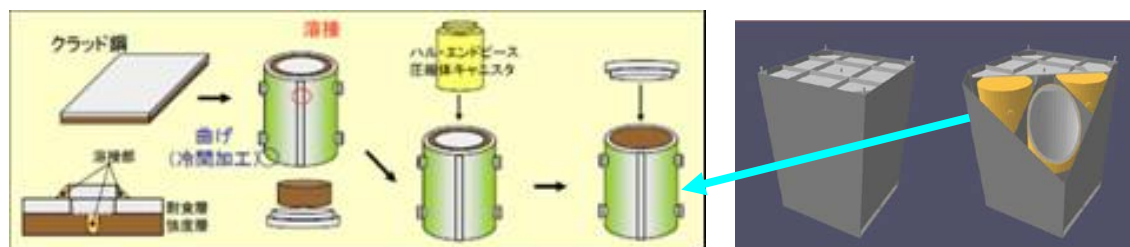
図 3－9 4 金属容器の製作方法
