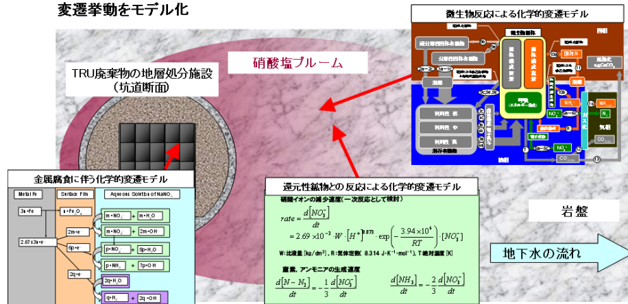
図 3-103. 硝酸塩化学変遷評価モデルの構成図
