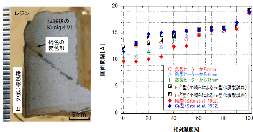
図3-32. ABM試験後試料の写真(左)及び試験後試料(鉄製ヒータから5、10、75mmの試料)とFe型・Na型・Ca型スメクタイトの底面間隔変化の比較(右)
