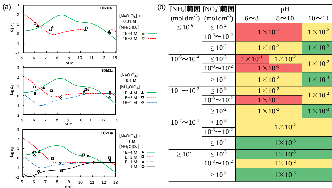
図 3-105. 核種の分配係数の推定結果の例 (a) Pd 分配係数のモデル化、(b) モデル化に基づいた推定値
