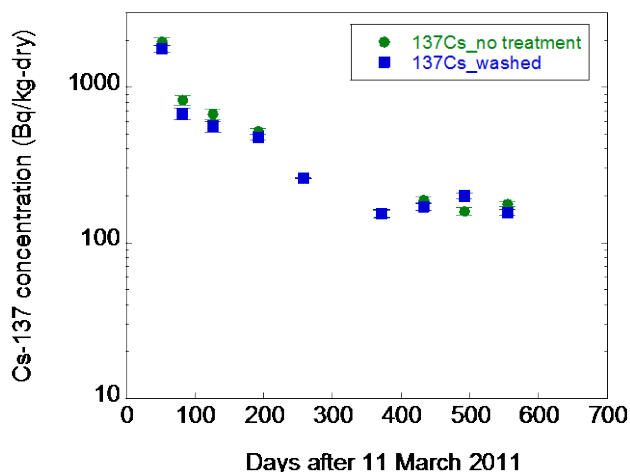
図 3－140. 植物葉中の Cs-137 濃度変化
