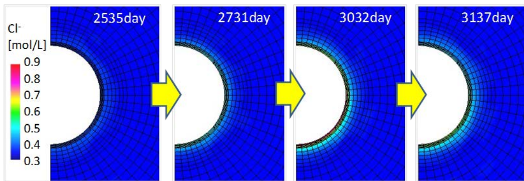
図 3－30 トンネル周辺岩盤の間隙水中の塩素イオン濃度の経時変化例
