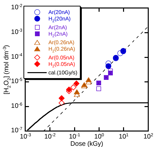
図 3－23. イオン照射試験による検証の例（Ar、 \text{H}_2 の雰囲気気条件）
