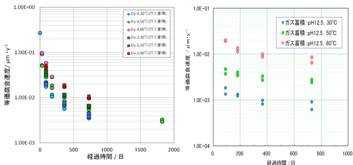
図 3-98. 高アルカリ・低酸素条件における腐食速度 （左：ジルカロイの腐食速度、右：ステンレス鋼の腐食速度）
