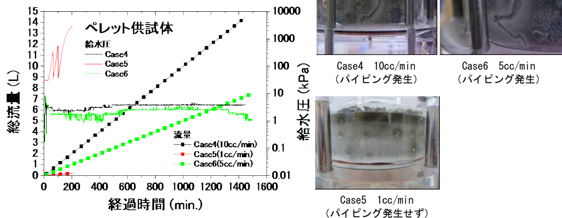
図 3-44. 人工バリア品質評価・緩衝材／ (ベントナイトペレット充填供試体のパイピング発生条件（流量）の取得試験）
