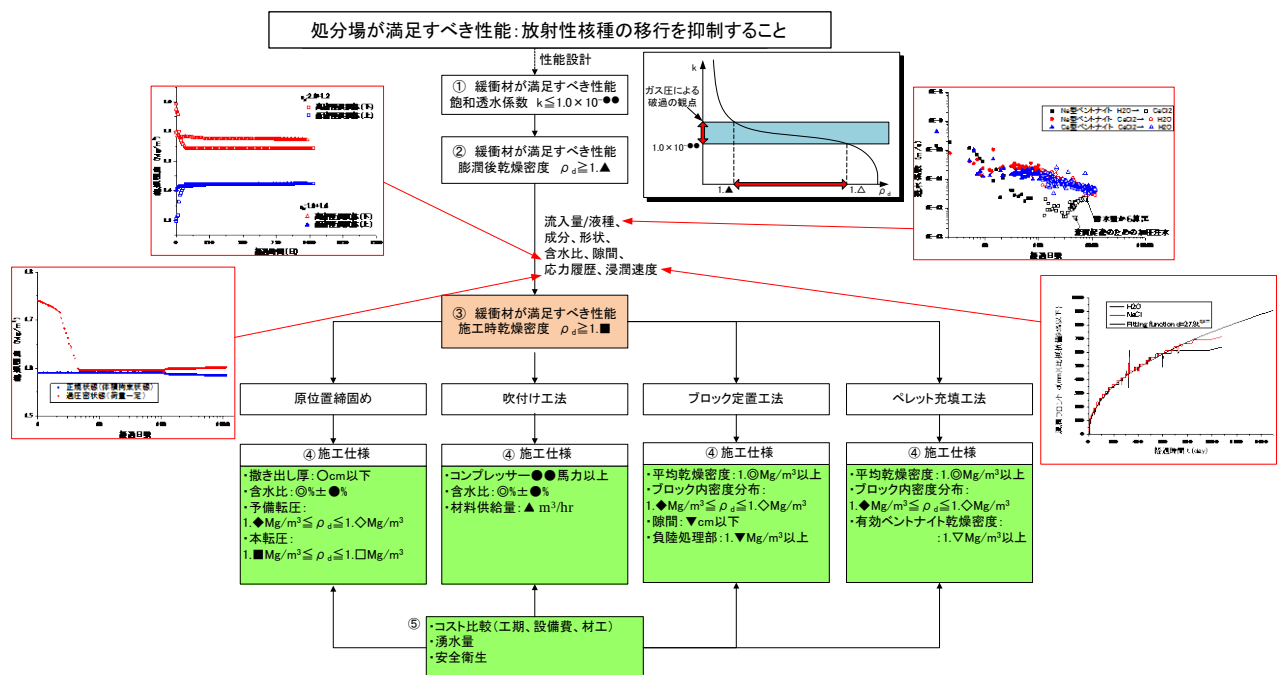
図 3-45. 人工バリア品質評価・緩衝材／ (緩衝材の設計・施工仕様設定のプロセス（案）)
