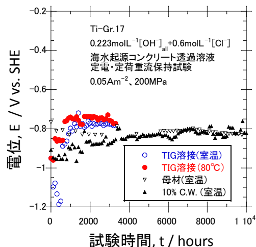
図 3－96． 定電流保持試験 (水素に起因する応力腐食割れ 感受性確認結果)
