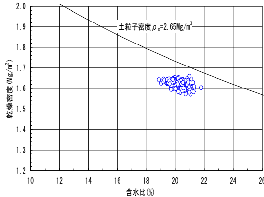
図 3-124. 含水比と乾燥密度の関係
