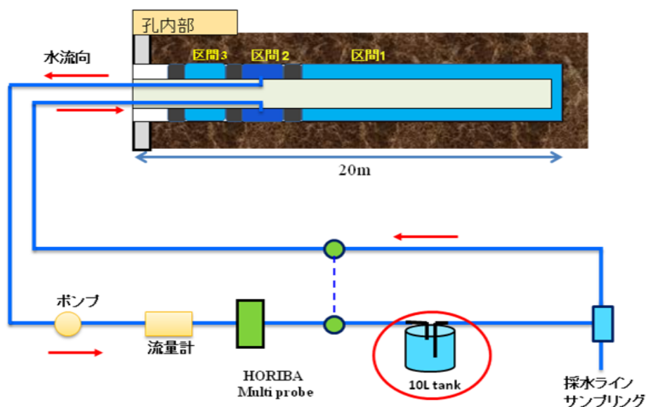
図3-27 酸化還元変化原位置試験手法
