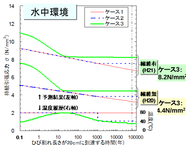
図 3－9 2. 長期ひび割れ進展評価結果
