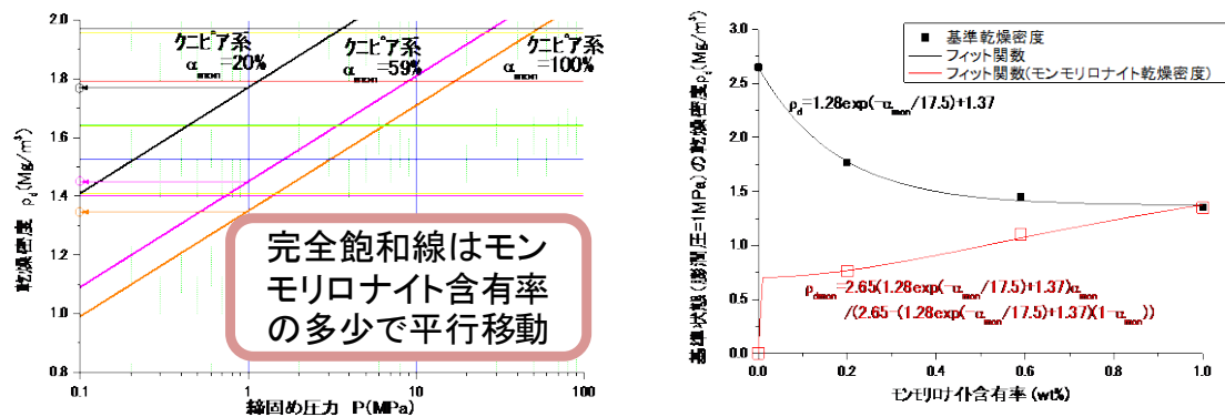
図 3-74. モンモリロナイト含有率の変化と力学特性変化
