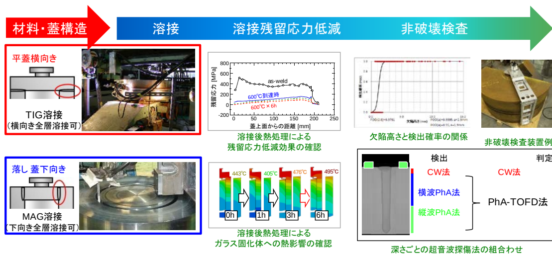
図 3-39. 遠隔操作技術高度化開発 (溶接・検査技術に関する成果の一例：オーバーパック溶接・検査システム案)
