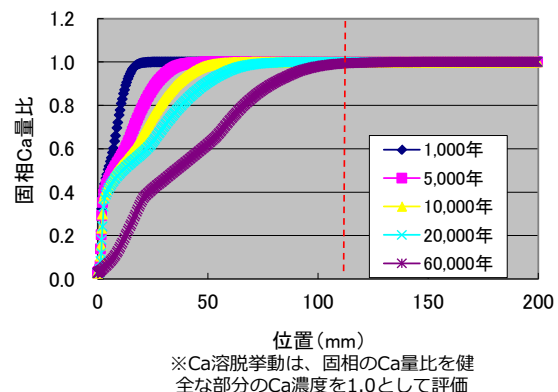
図3-91. Ca の溶解の予測結果
