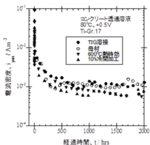
図 3－95． 定電位保持試験 (不動態健全性確認結果)
