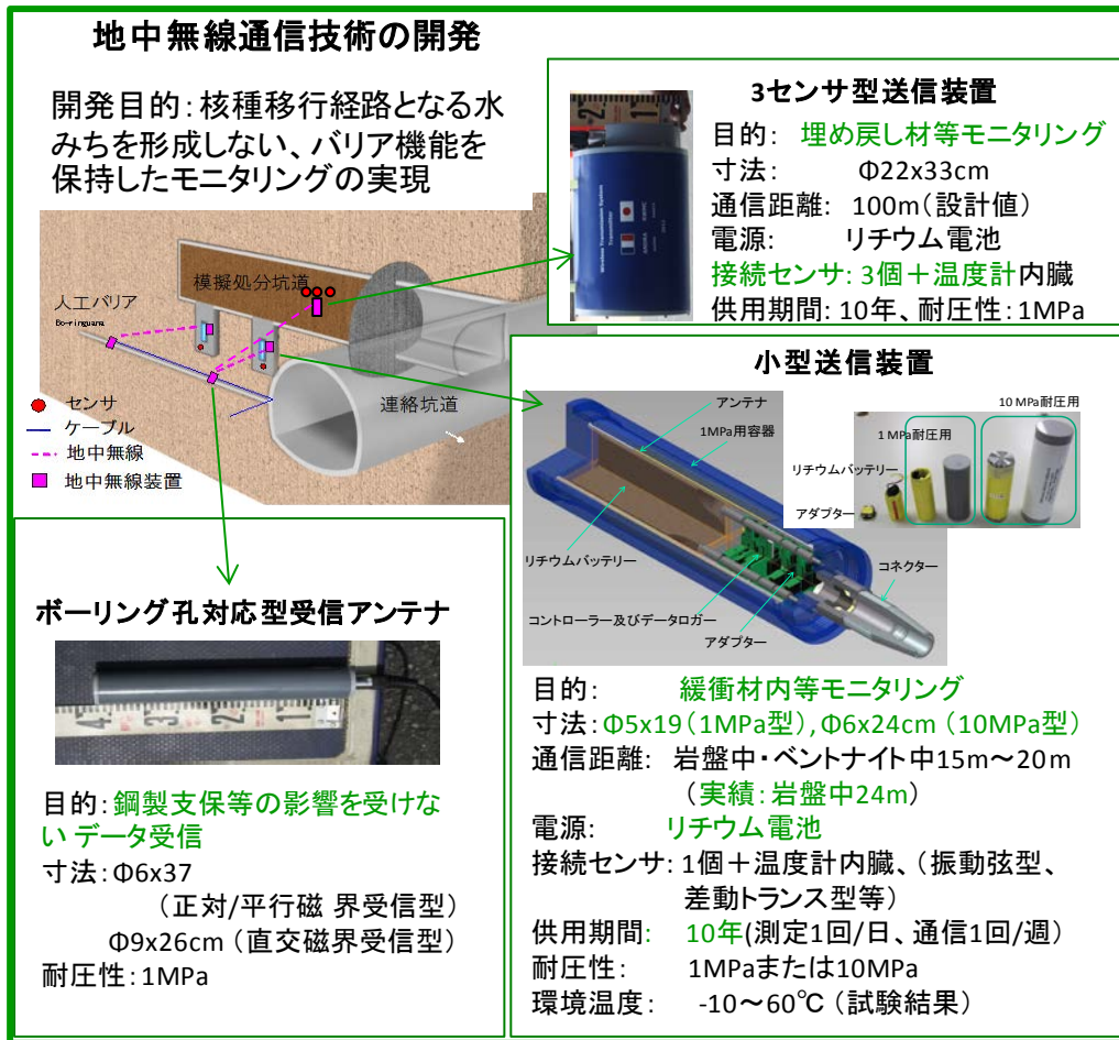
図3-47. モニタリング技術・中核的な要素技術の成果の一例／ (地中無線通信技術の開発：開発した小型地中無線送信装置等及び想定される使用法)
