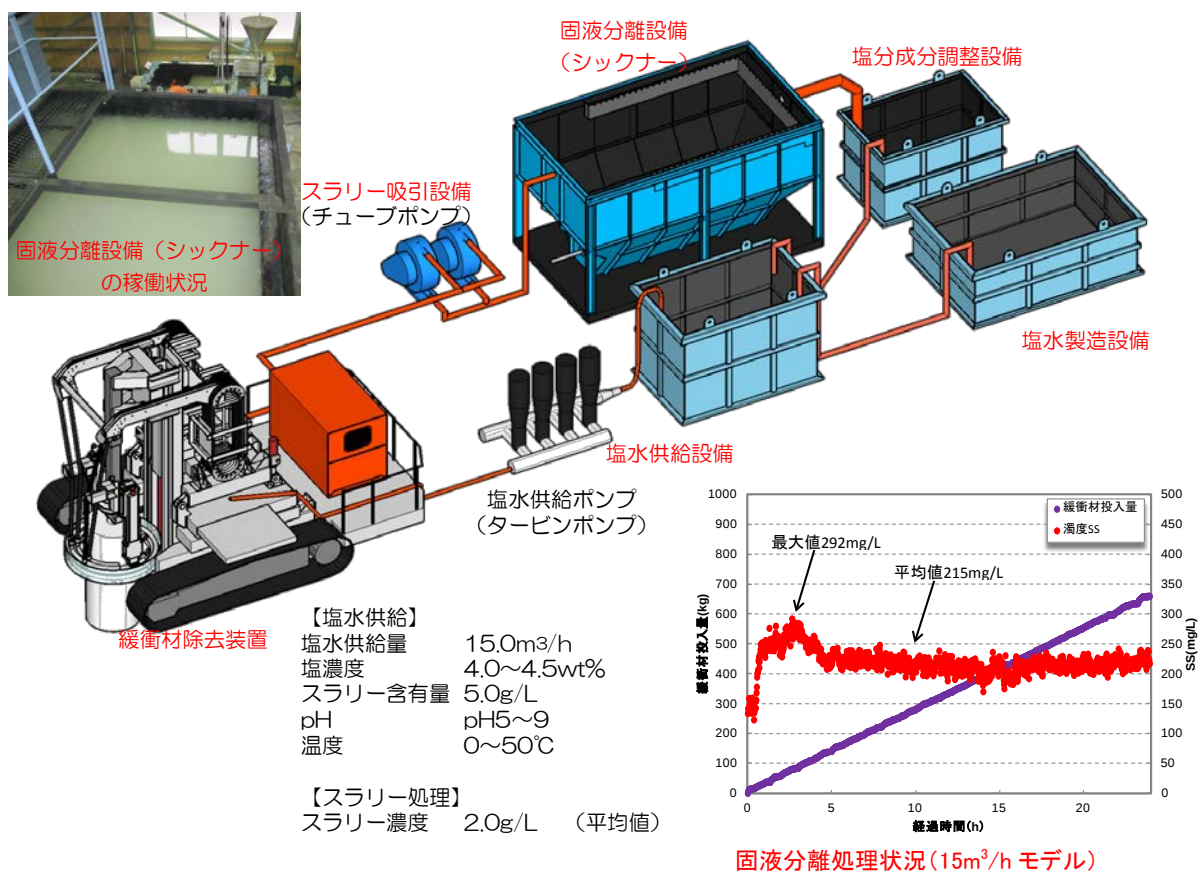
図 3 - 5 5 . 塩水リユース設備の構成と試験状況
