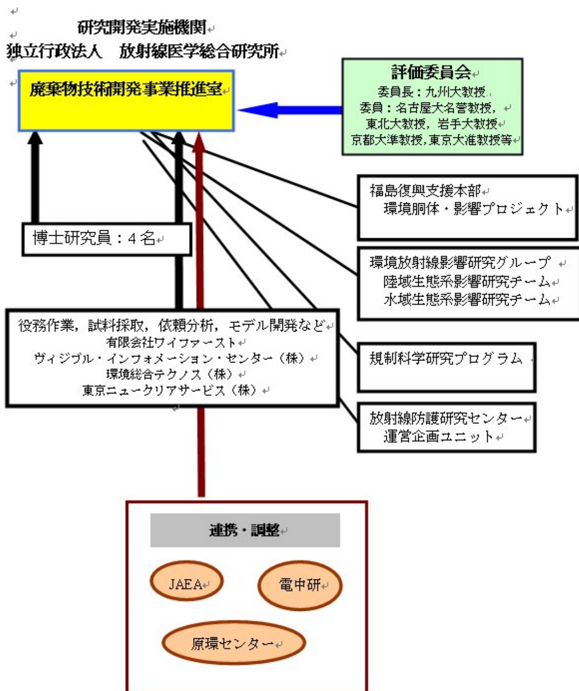
図 3－1 4 2．研究開発実施体制（放射性核種生物圏移行評価高度化調査）
