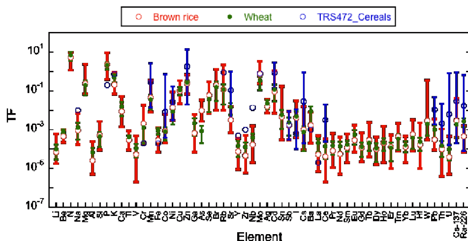
図 3-138. 本調査で得られた TF 値と IAEA の TF 値
