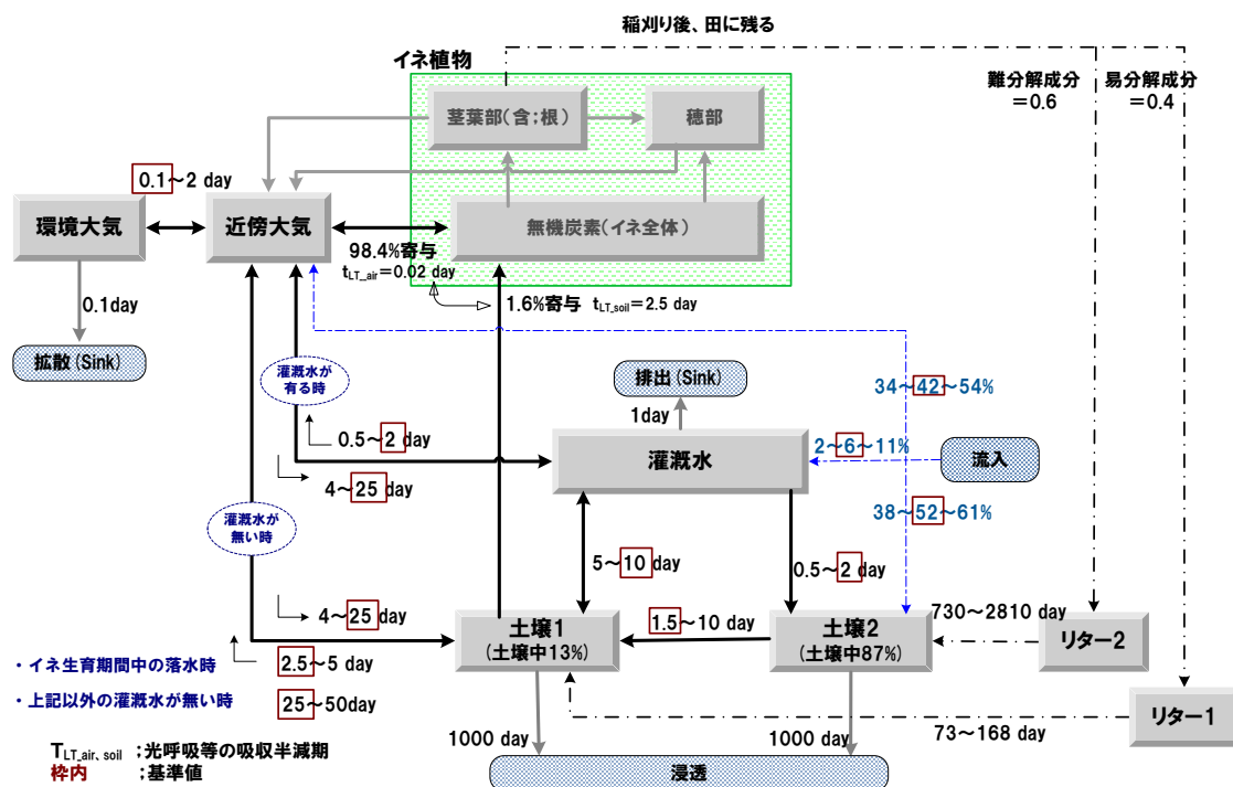
図 3-135. 水稻移行モデルと移行半減期 本調査および文献調査により得られたデータを用いて 構築した水稻全体モデルにおける ^{14}\text{C} の移行半減期を決定
