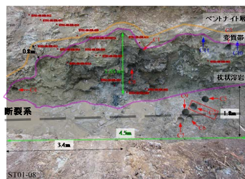
図 3－132．Saile 鉱山のベントナイトー枕状溶岩の断面と変質部（Bleached Zone）
