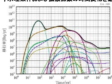
図 3-76. 人工バリアでの核種移行計算の結果
