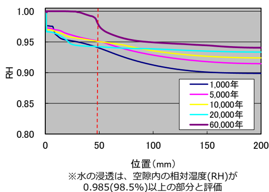
図3-90. 水の浸透挙動の予測結果
