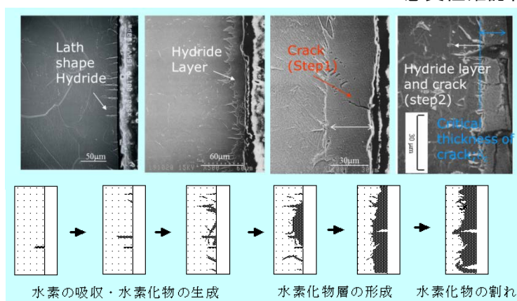
図 3－97． 水素化物層の観察結果と生成・割れによる亀裂進展モデル
