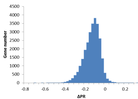
図(1)-3-6 植物の生長における翻訳状態変化 (ΔPR 値)
