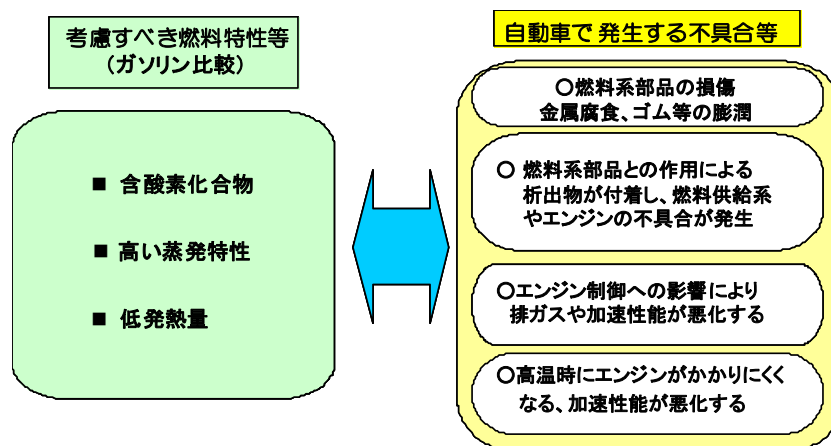
図 3-1-1 エタノールのガソリンへの混合時の特徴と課題
