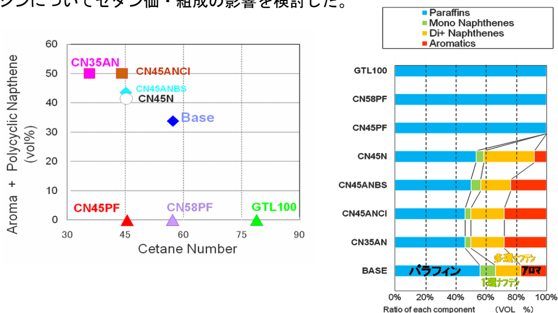
図 3-1-13 評価燃料の性状と組成
