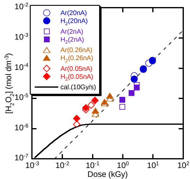
図 3－23. イオン照射試験による検証の例（Ar、H 2 の雰囲気条件）
