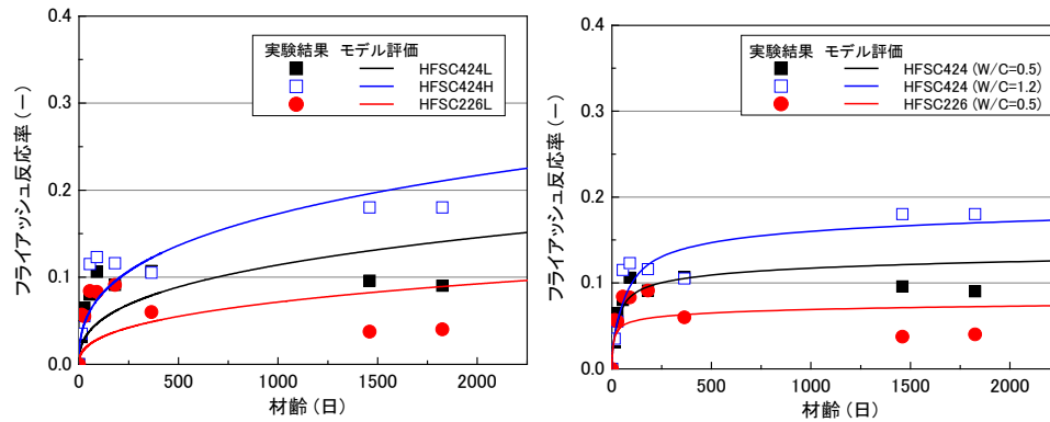
(図3-100) Shrinkage Coreモデルによるフライアッシュ反応率の評価結果 (左図：既存の Shrinkage Coreモデル、右図：改良後の Shrinkage Coreモデルでの評価)
