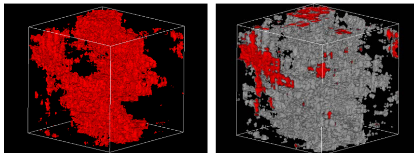
(赤色: 空隙、灰色: ケイ酸カルシウム水和物(C-S-H)) 図3-68. 変質に伴う物質移行特性(拡散係数)算定手法で使用するセメント水和物と空隙構造の三次元モデル
