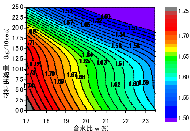
図 3-125. 吹付けベントナイトの含水比—供給量—乾燥密度の関係
