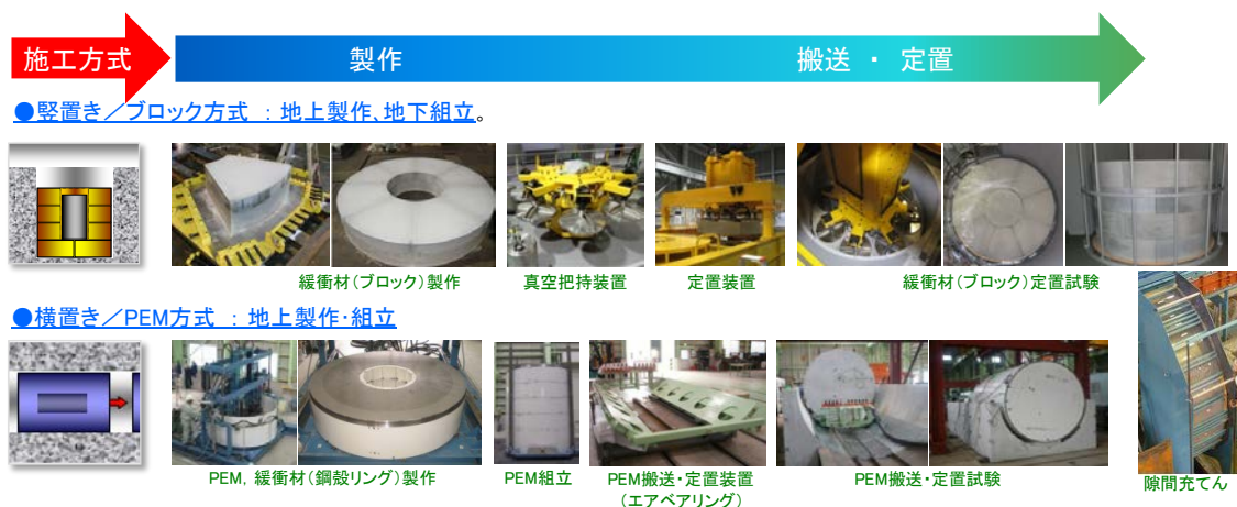
図 3 - 4 0 遠隔操作技術高度化開発／ (搬送・定置技術に関する成果の一例：緩衝材の搬送・定置システム案)
