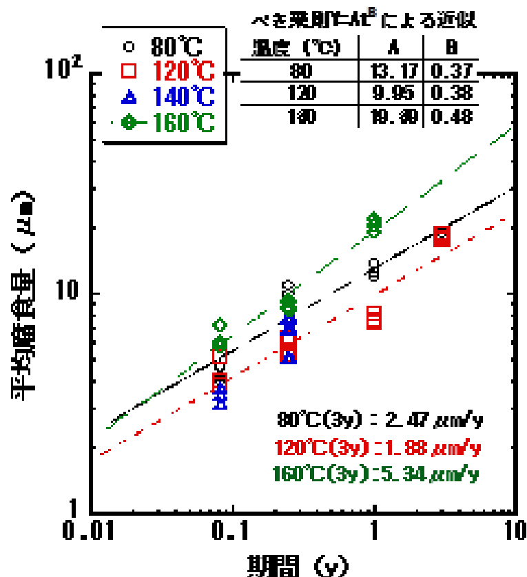
図 3-31 全面腐食挙動（還元性）試験結果
