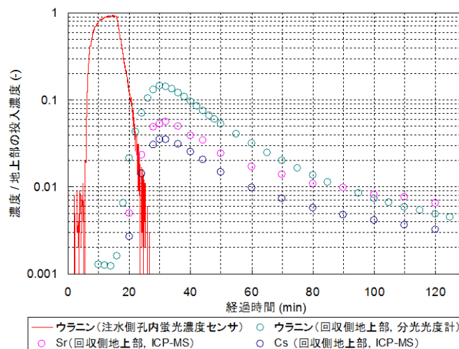
(b) トレーサ試験の注水側と回収側の濃度変化
