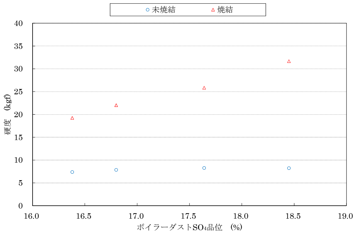
図 3-57 \text{ZnSO}_4 が焼結に及ぼす影響（添加）
