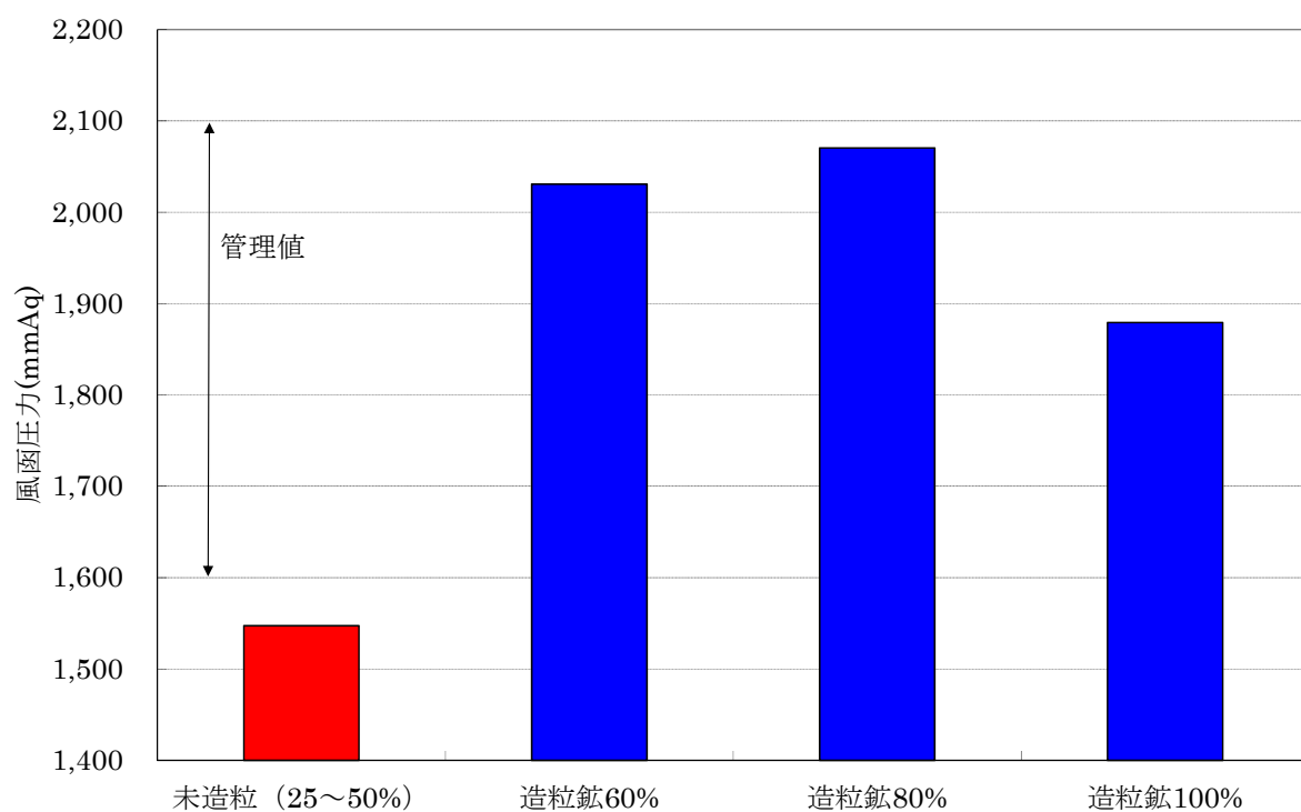
图 3-26 風函圧力
