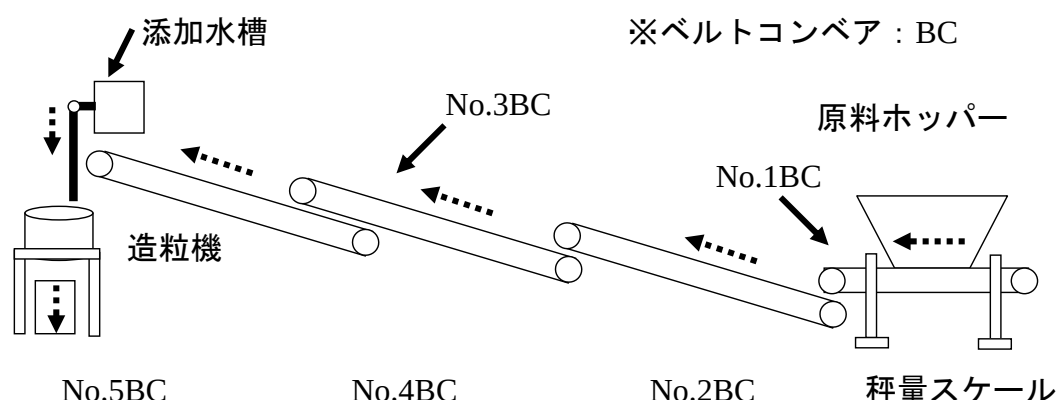
図 3-30 造粒鉱作成試験装置概略図
