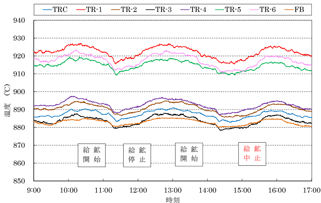
図 3-32 造粒鋇供用時の温度変化 (1 日目)
