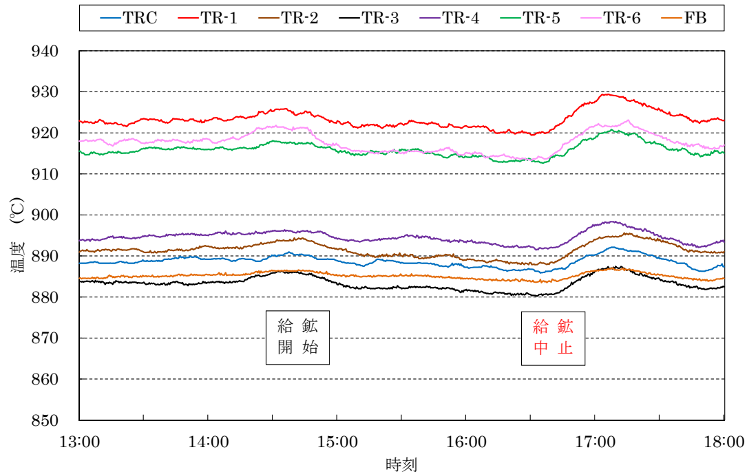
図 3-34 造粒鋳供用時の温度変化
