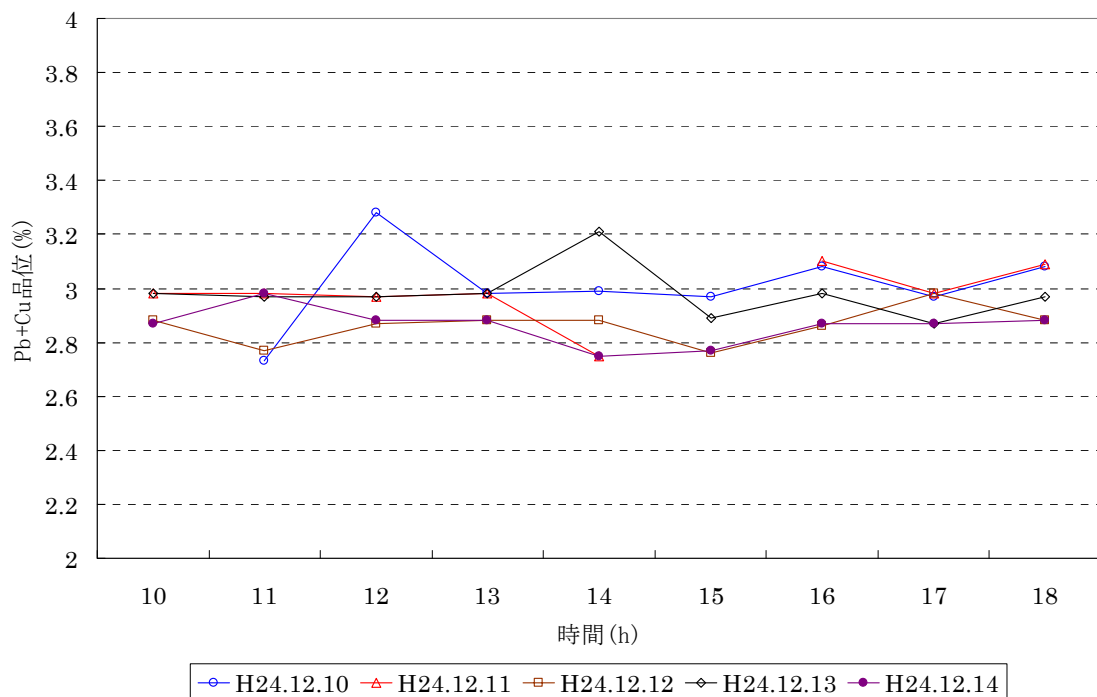
図 3-29 混合後精鉱の Pb+Cu 品位推移
