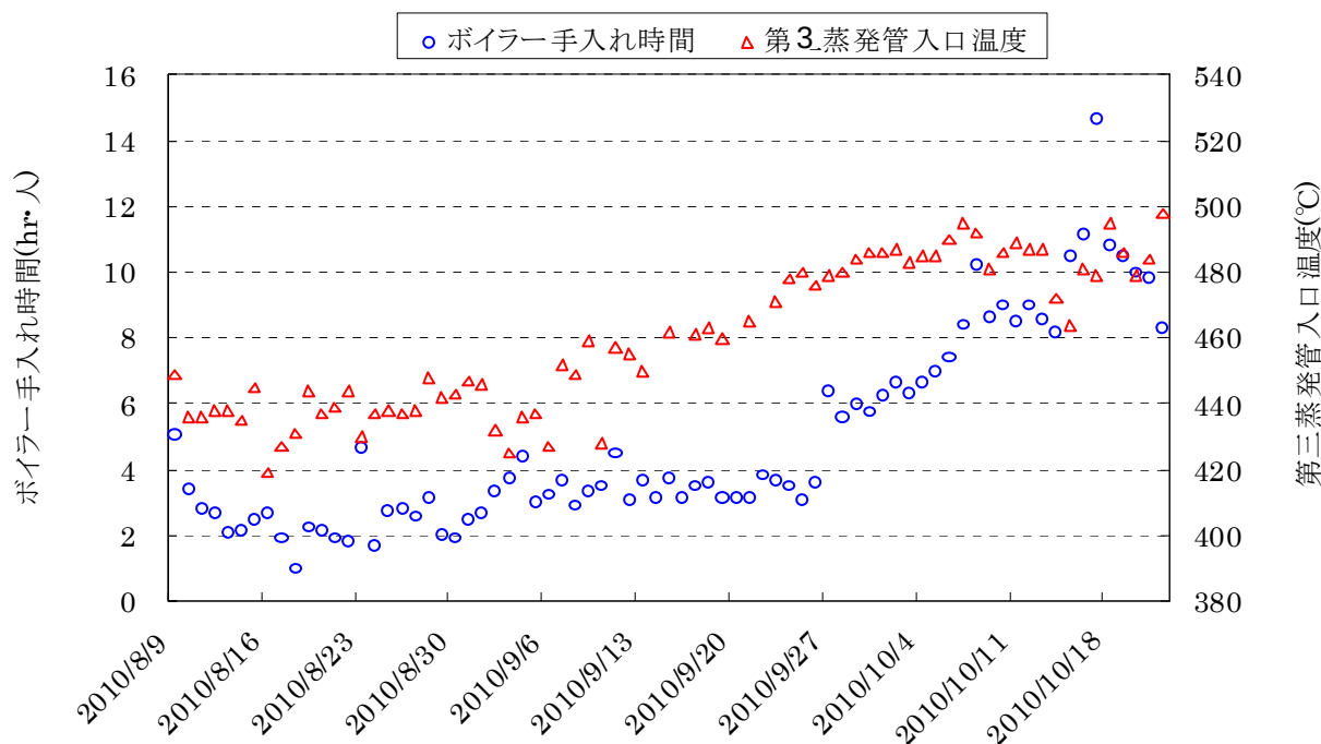
図 3-48 微粉鉬供用試験時のボイラー手入れ時間、第 3 蒸発管入口温度の推移
