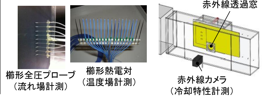
図3 計測装置
