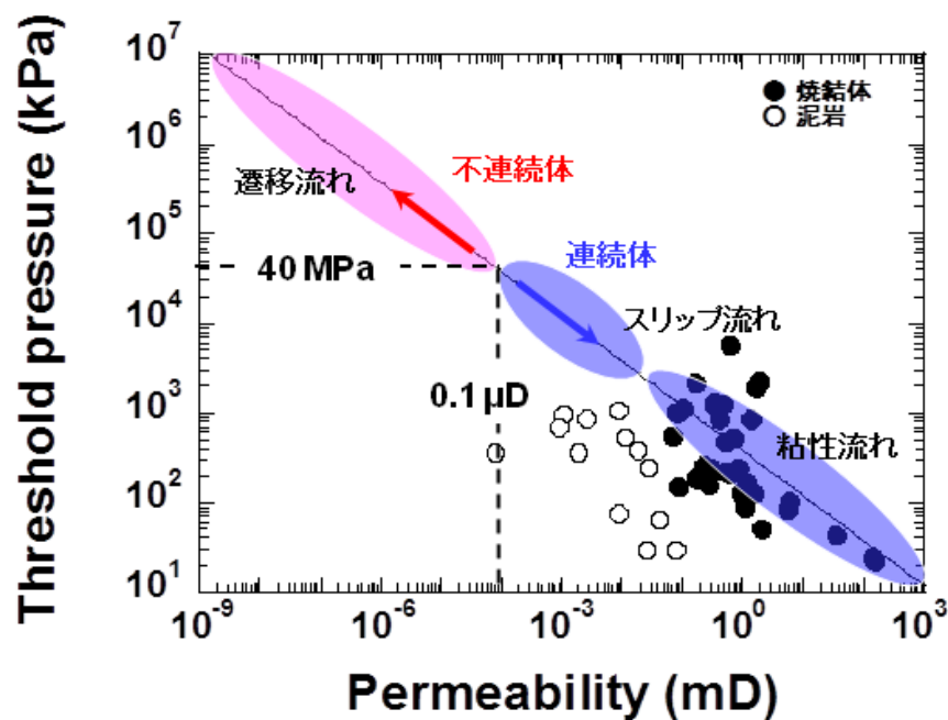
図 3.I.1-12 焼結体と岩石におけるスレッシュホールド圧－浸透率の相関性の比較
