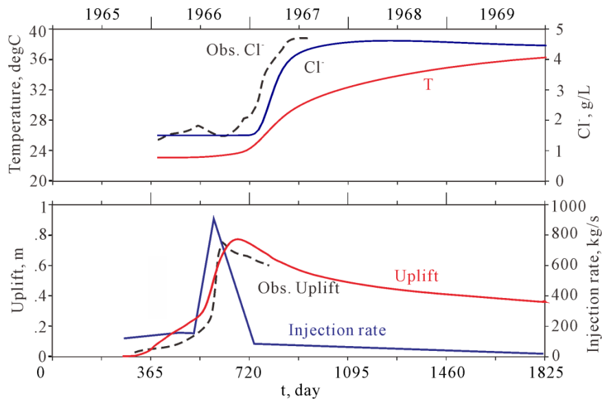
図 3.I.2-40 観測された最大地表隆起量と \text{Cl}^- 濃度 (modified from Noguchi et al., 1969)、断層ゾーン細分割モデルを用いて計算された最大垂直変位と \text{Cl}^- 濃度、および計算に用いた地下からの水の圧入量。
