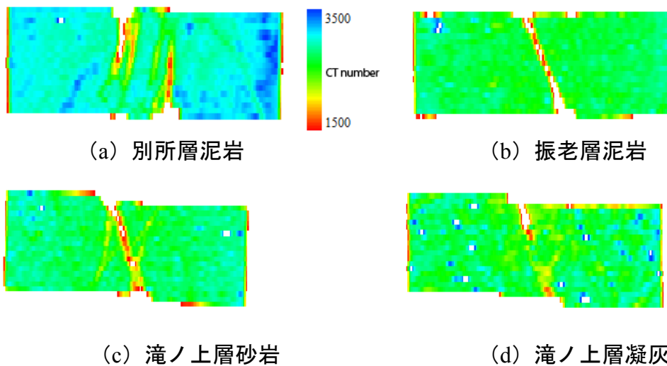
図 3.I.2-42 X線CTによる岩石の内部組織観察の結果(3D解析にはGeoTaosのソフトウェアを使用)
