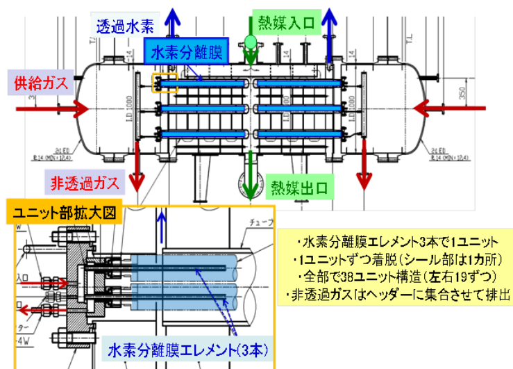
200N m³/h 級熱交換器一体型分離膜モジュール
