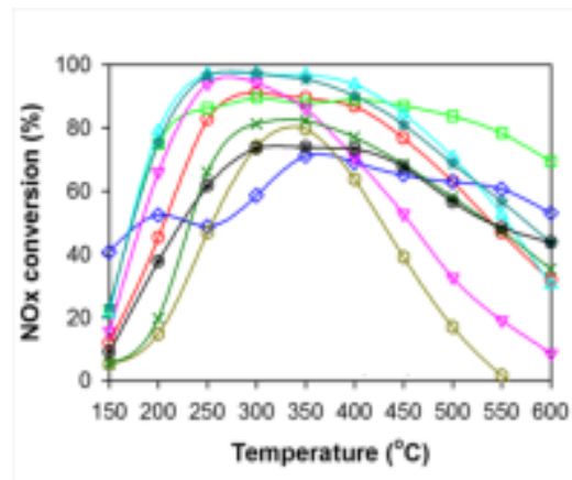
様々な銅ゼオライト触媒の NOx 浄化特性 (カタログ掲載性能の一項目)
