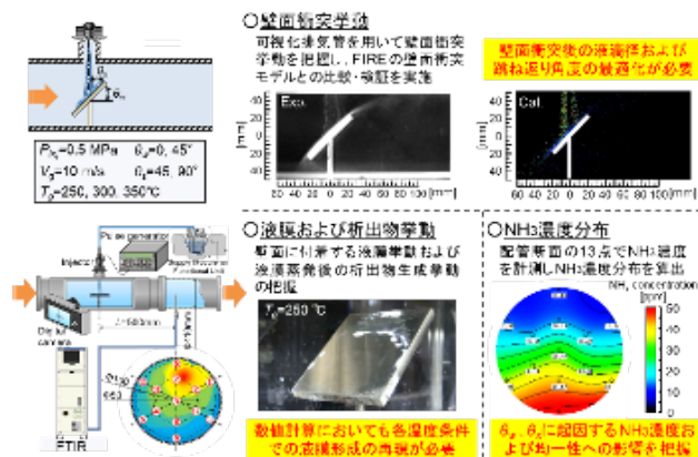
尿素の壁面衝突噴霧の現象解明
