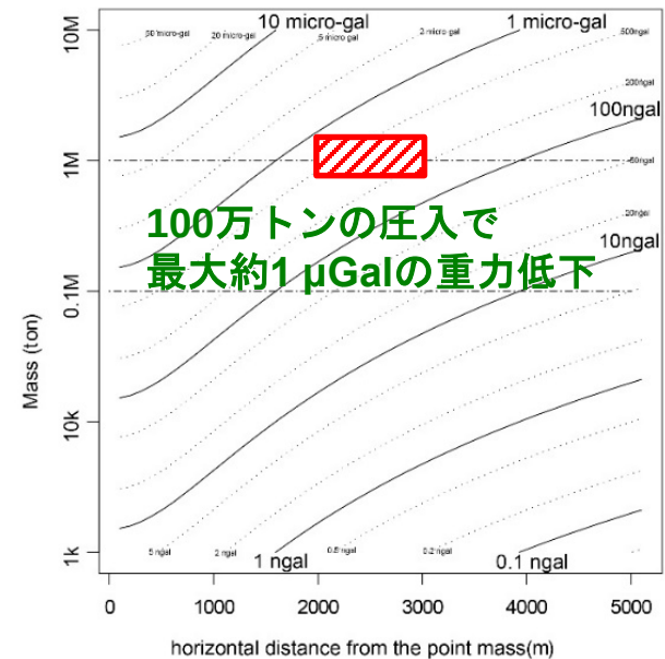
深度1kmの点質量変化によって地表に生じる重力変化
