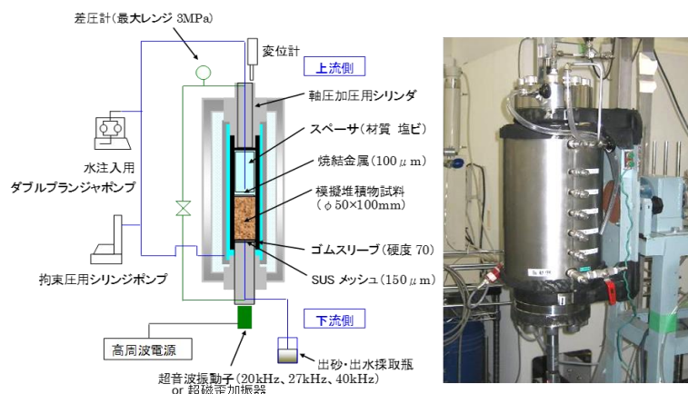
図 小型実験装置 (今回実験で使用) (試料寸法: \phi 5\text{cm} \times 10\text{cm} 、1次元流れの透水実験用)
