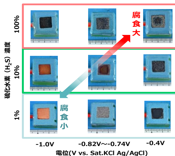
図2. A — 43 銅の腐食挙動への硫化物濃度と酸化還元性*の影響（硫化銅の皮膜形成の確認） *：電気化学試験の電位として設定
