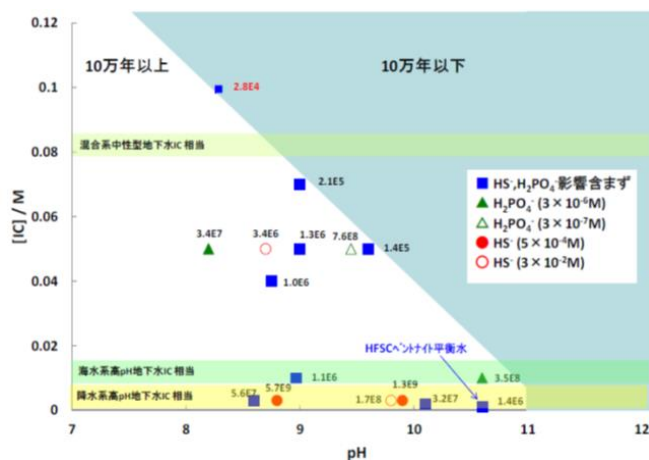
図2. A — 31 BPI ガラス固化体の寿命評価
