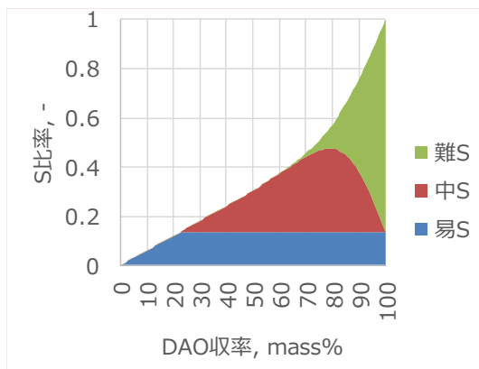
図 4-21 DAO 収率と硫黄タイプの推移
