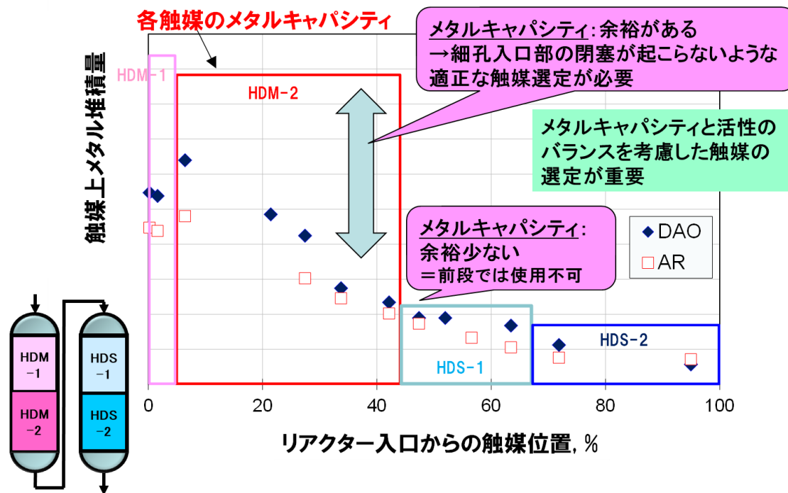
図 4-32 DAO 処理に望まれる触媒機能
