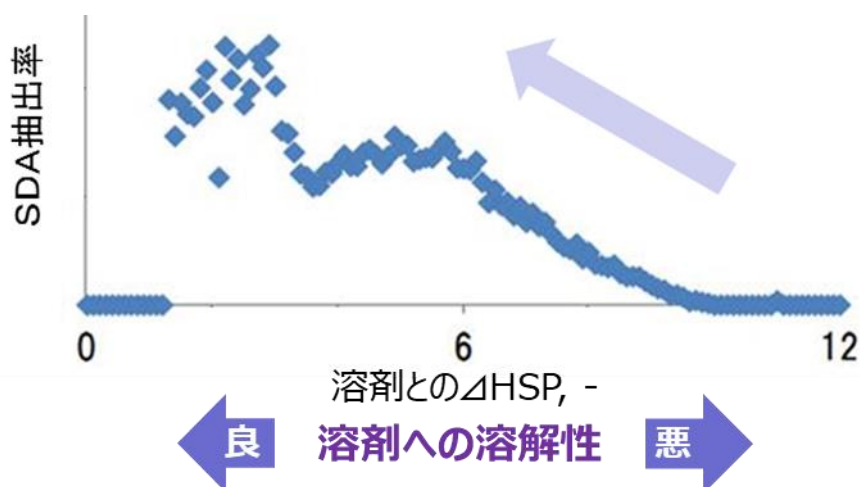
図4-18 SDA原料分子の \Delta HSP とSDA抽出率の相関
