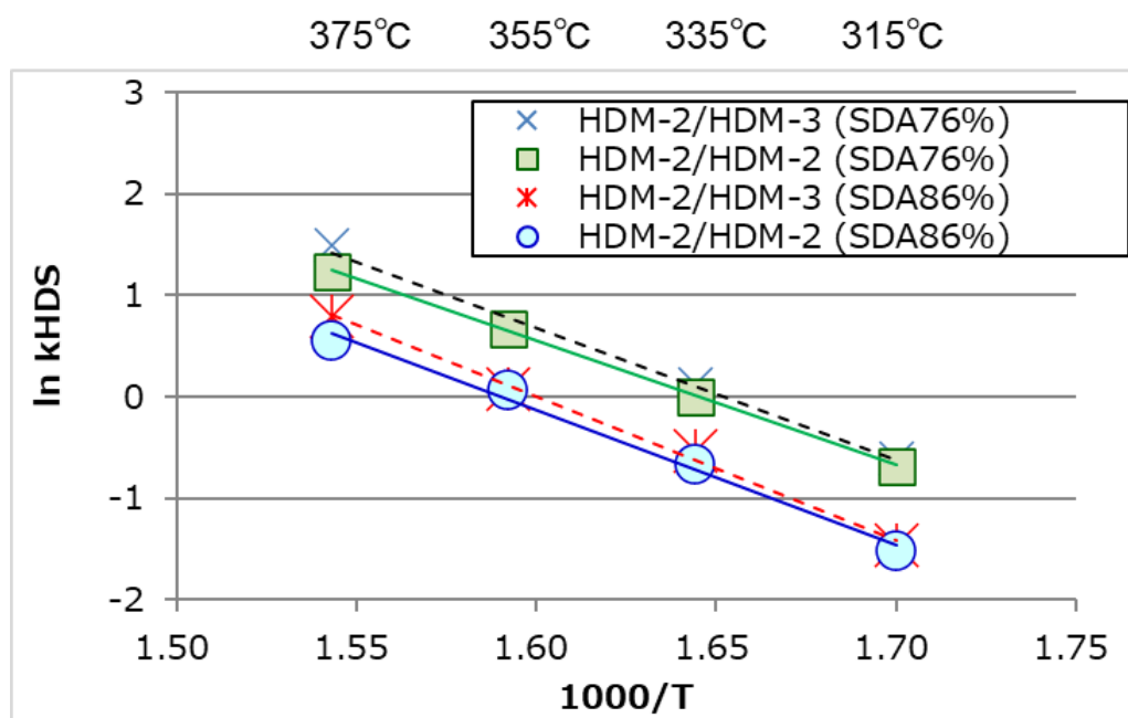
図４－３８ 抽出率の異なるＤＡＯの反応性比較（ＨＤＳ反応）
