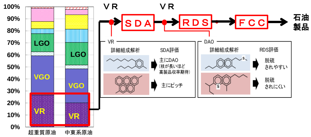
図 4－9 詳細組成構造解析のイメージ
