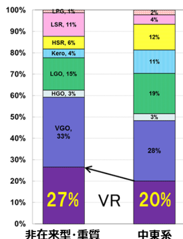
図４－８ 重質原油と中東系原油の収率比較
