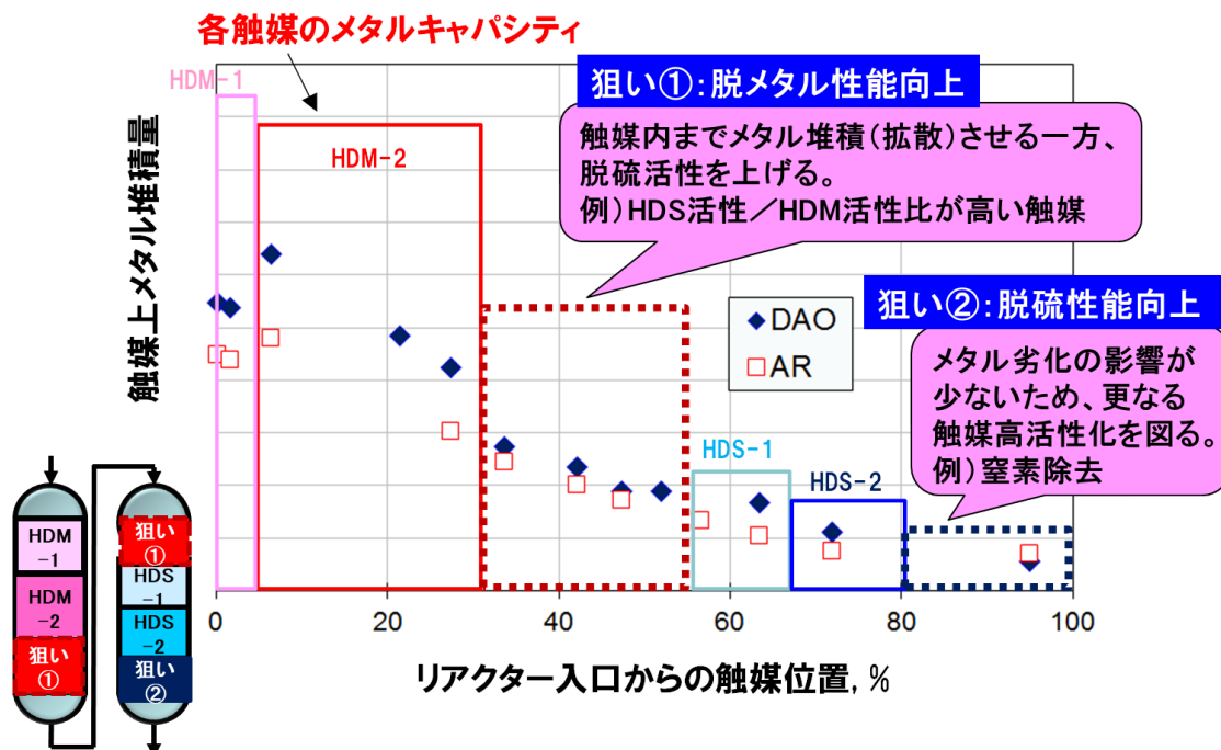
図 4-33 DAO 処理用触媒システムのコンセプト
