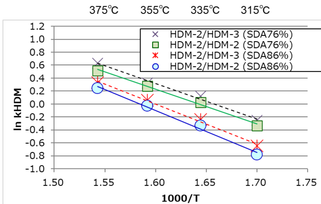
図４－３９ 抽出率の異なるＤＡＯの反応性比較（ＨＤＭ反応）
