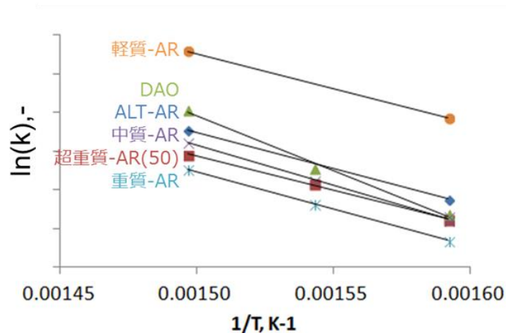
図 4 - 1 5 R D S 反応性結果
