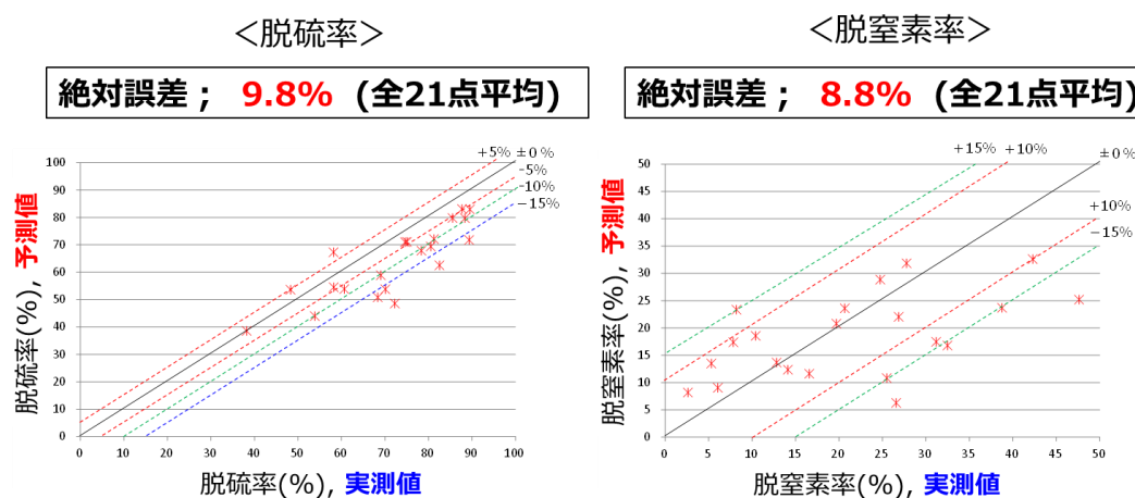
図6-2 AR の脱硫率及び脱窒素率の予測モデル検証結果
