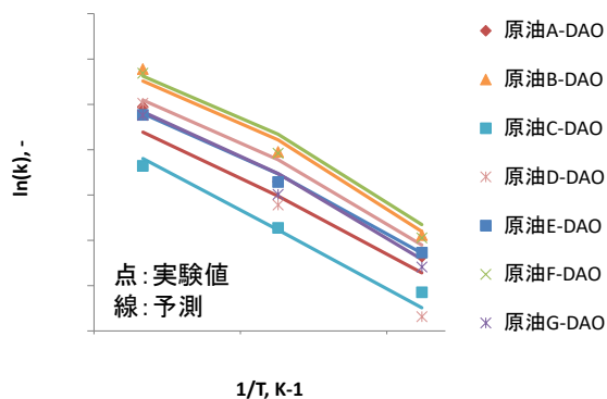
図 4-22 DAO の RDS 脱硫反応性予測
