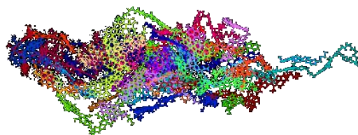
図6-17 分子シミュレーション技術によるアスファルテン凝集体のイメージ
