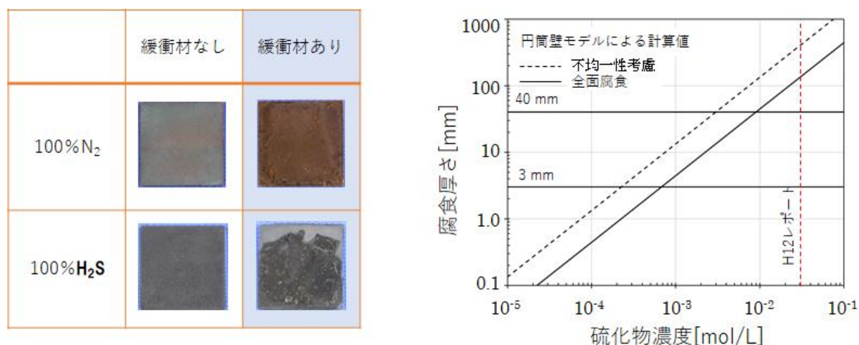
図 2B-38 腐食評価の成果の例 (左：浸漬試験後の試験片外観 (試験期間 100 日)、右：長期腐食量の評価結果の例)
