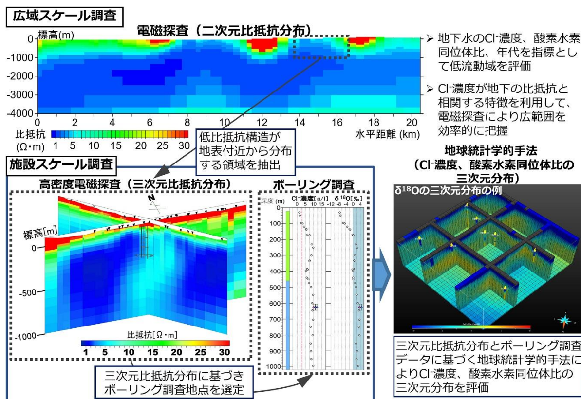
図 2B-6 電磁探査とボーリング調査を組み合わせた低流動域の三次元分布の評価例
