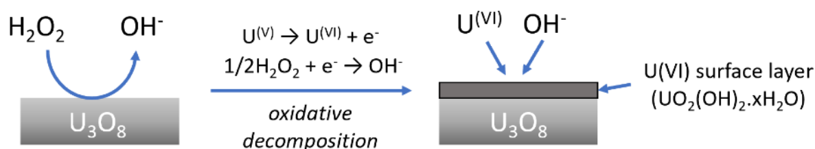
図 2B-37 \text{U}_3\text{O}_8 への固相析出による \text{H}_2\text{O}_2 反応経路の変化の概念 25)
