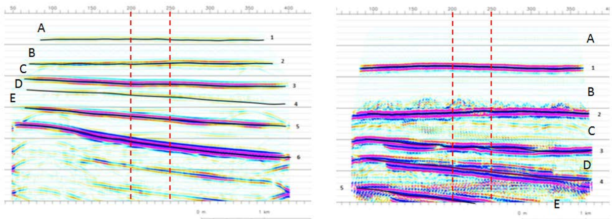
図 3.I.1-5 苫小牧沖での合成弾性波探査データによる P 波重合記録（右）と PS 変換波重合記録（左）。アルファベットは仮定した同一地層を示す。
