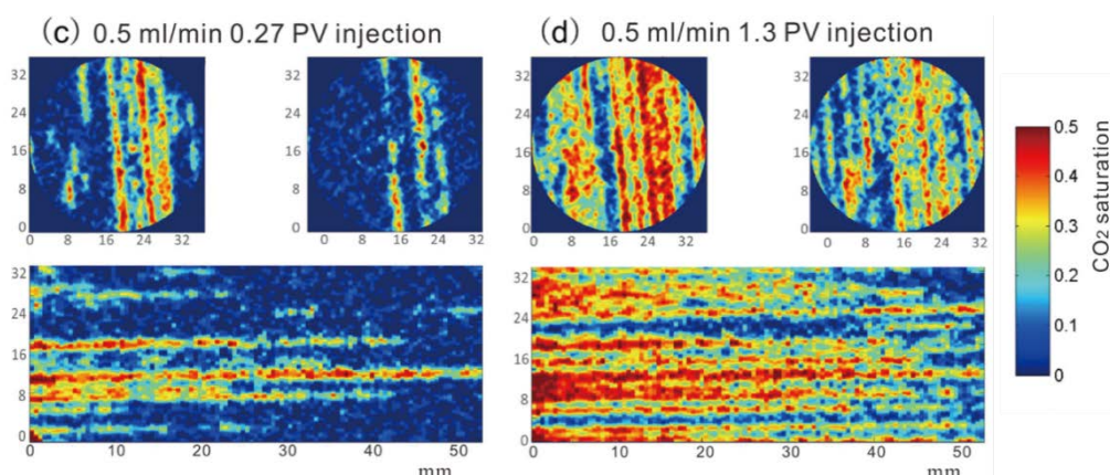
図 3.I.2-16 ドレネージにおける \text{CO}_2 飽和度分布
