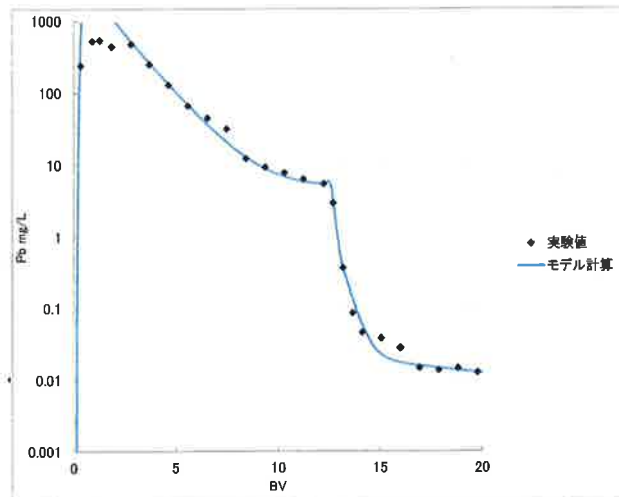
カラムテスト①の数値モデル化
