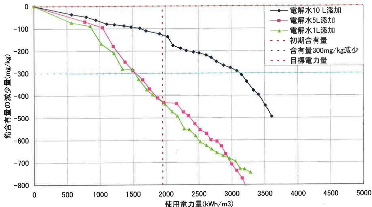
図 3-1-2(3)-7-6. 電解水添加の影響
