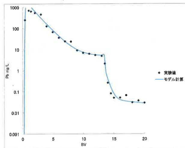
カラムテスト③の数値モデル化
