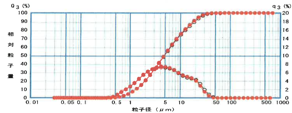
図-3-1-2(3)-5. 笠岡粘土の粒度分布
