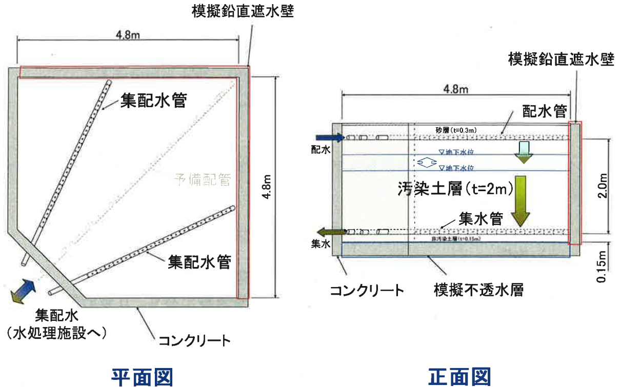
図 3-1-2(2)-3 地上土槽 概要図
