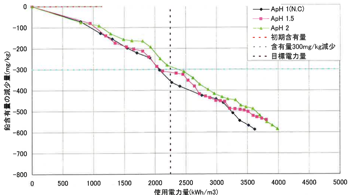
図 3-1-2(3)-7-4. 電解液 pH、EC の影響
