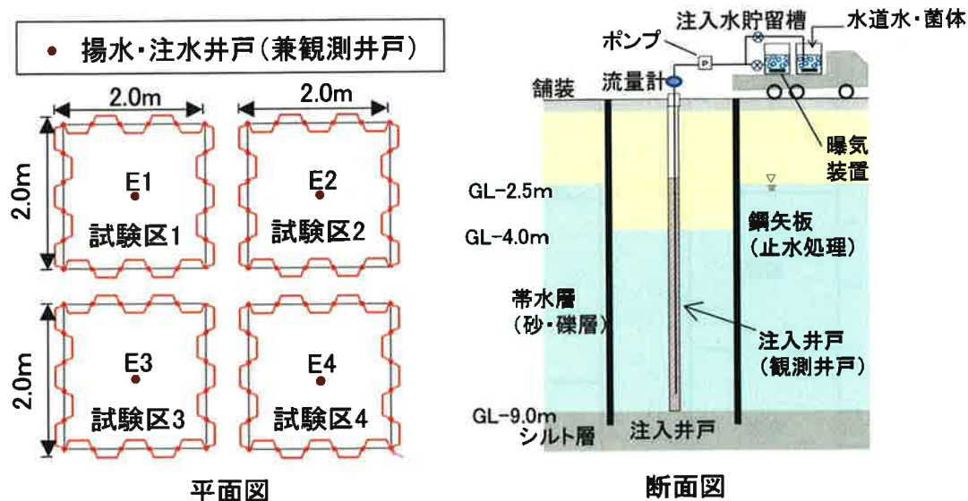
図 3-1-2(4)-60. 実証試験サイトの概略図
