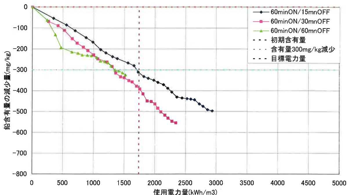
図 3-1-2(3)-7-5. 印加電圧パルスの影響
