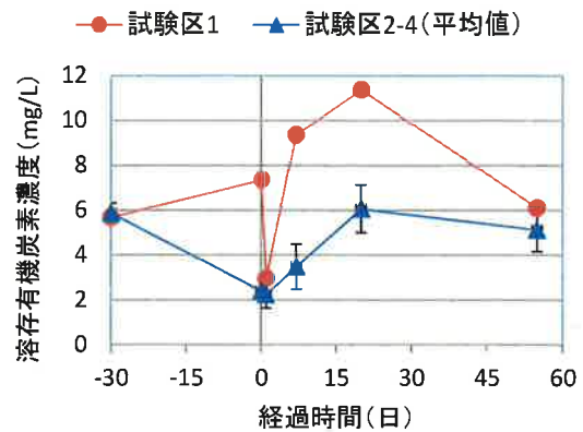
図 3-1-2 (4)-66. DOC の推移
