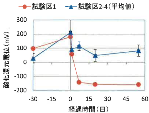
図 3-1-2 (4)-65. ORP の推移
