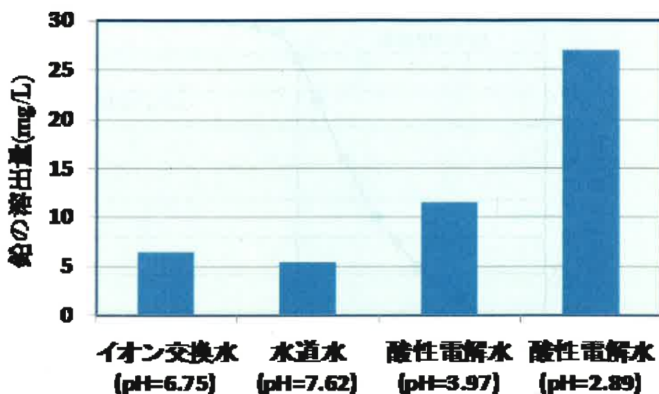
図 3-1-2(3)-3-3. 異なる溶媒による鉛の溶出特性比較
