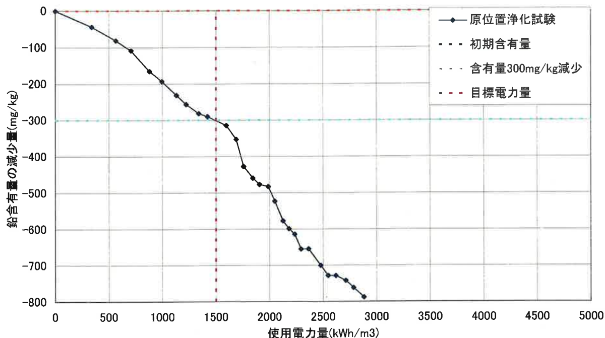
図 3-1-2(3)-10-1. 原位置実証試験結果
