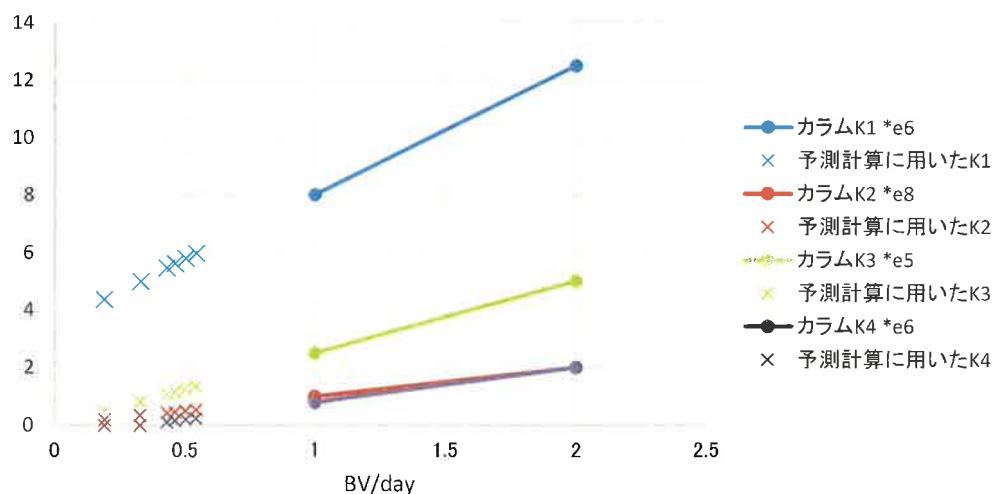
図-3-1-2(2)-26 地上土槽モデルのシミュレーション計算に用いる速度定数の
