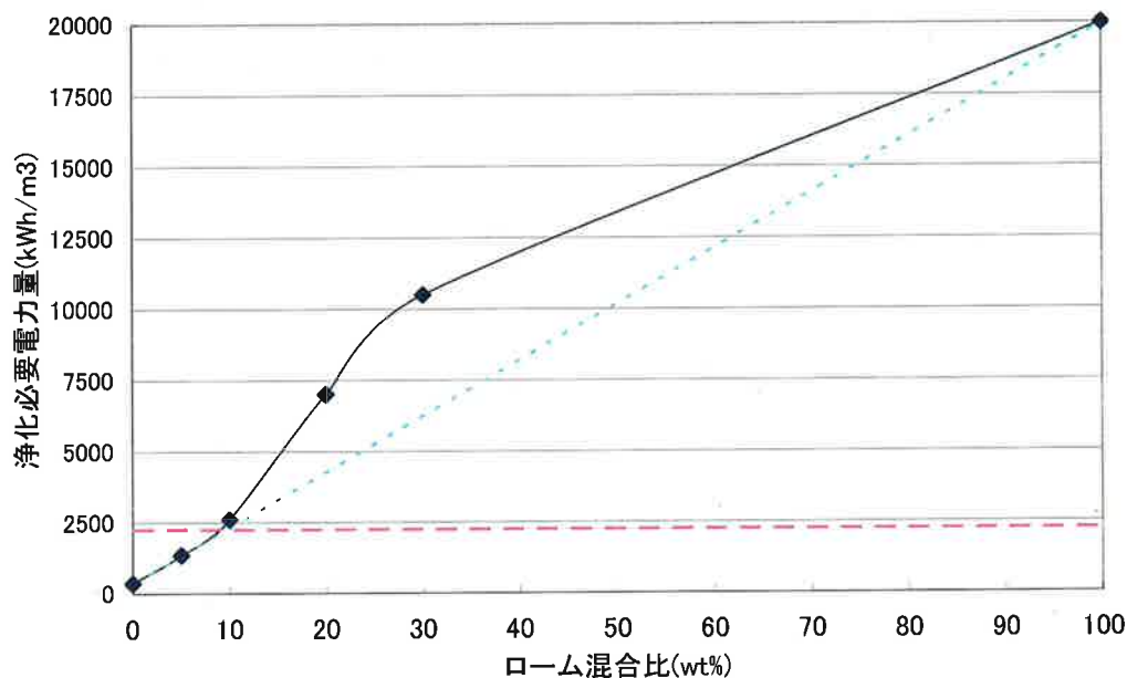
図 3-1-2(3)-14. 砂-ローム混合比対する浄化電力量
