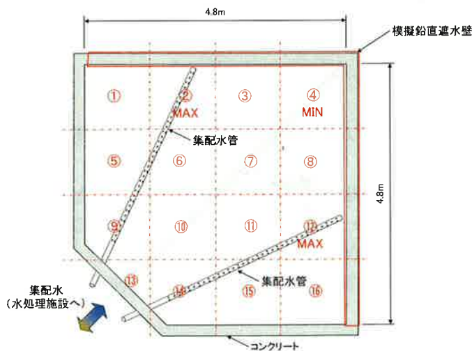
図-3-1-2(2)-27 ブロック分けと解析結果（流速）
