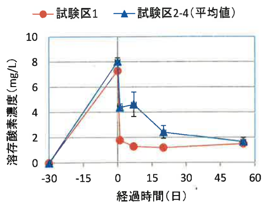
図 3-1-2(4)-64. DO の推移
