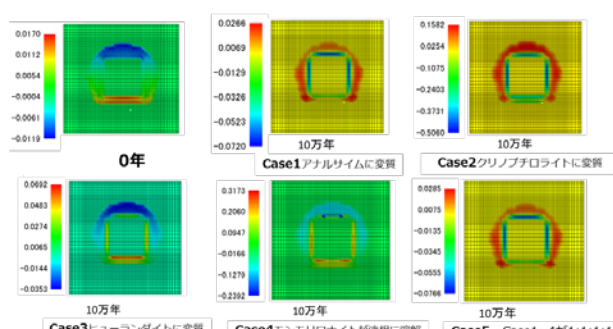
改良した水理-力学-化学連成解析によって予測した10万年後の処分場内の応力分布(化学変質による生成二次鉱物の違いによる応力分布の差(赤は圧縮状態(高密度)を示す))。
