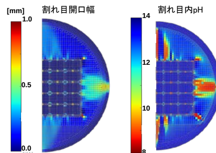
図2 複合現象評価モデルを用いた解析例 (TRU廃棄物処分坑道断面におけるセメント埋め戻し材中の、8,000年経過時の(a)割れ目開口幅及び(b)割れ目内間隙水のpH)
