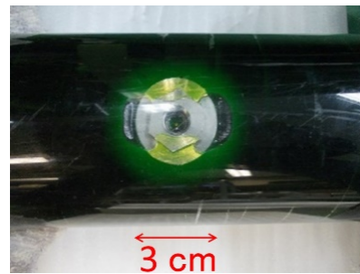
(b) アクリル管をボーリング孔に 見立ててウラニンを注入した
