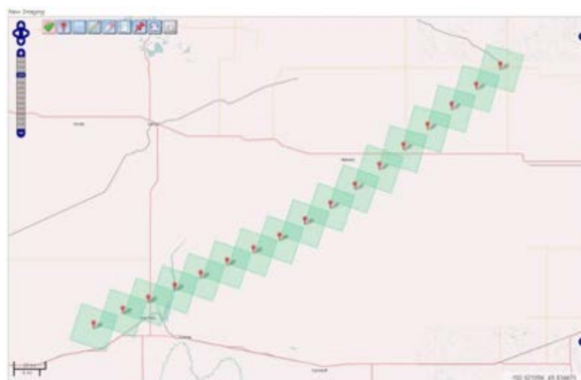
図 2.2.2-4 スナップショットモード撮像のフットプリント
