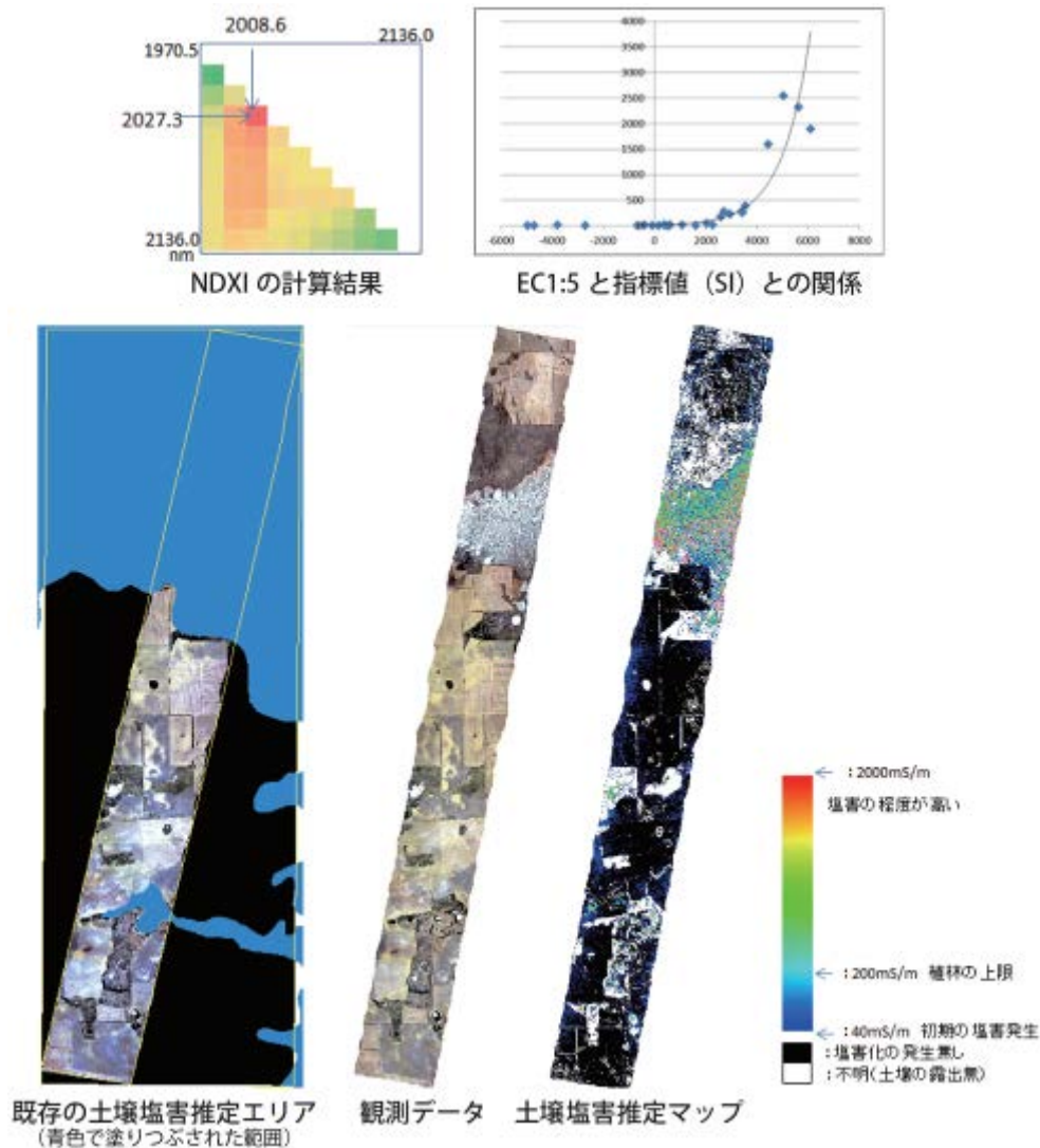
図 18 土壌塩害マップ
