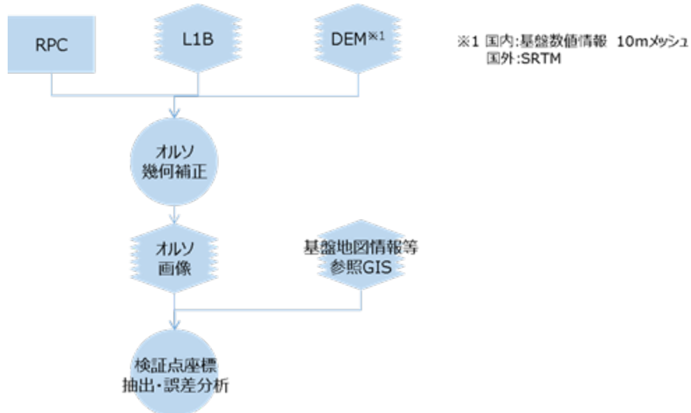
図 3.3.2-2 オルソ画像処理のながれ
