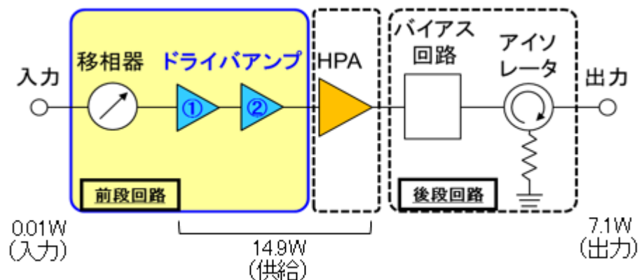
【HPA モジュール概略ブロック図】
