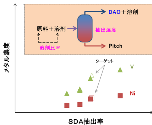
図4 SDAプロセスにおける運転条件の
