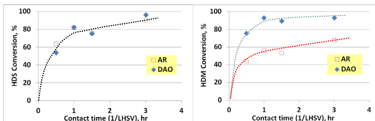
図5 ARとDAOの反応性比較
