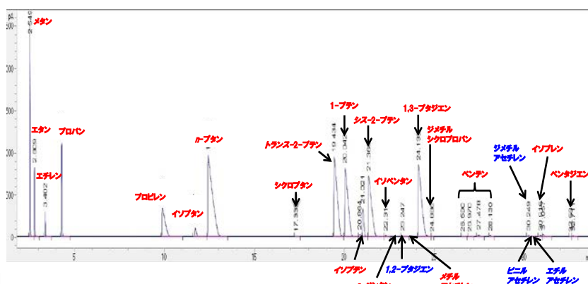
図9 反応器(2段反応)出口ガスの分析結果例
