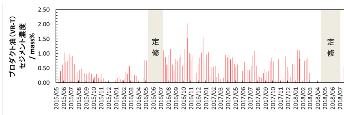
図 3 セジメント濃度の推移
