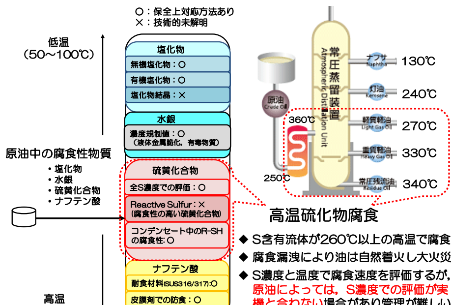
図1 劣質原油の腐食性物質と現状の技術・保全上対応方法
