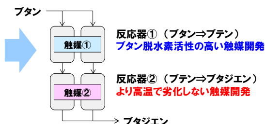
図5 ブタジエン収率向上のためのコンセプト
