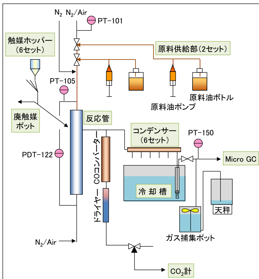
図 6 : DSAR 反応性評価装置
