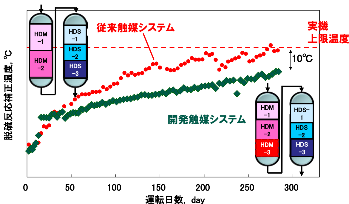
図8 市販触媒の性能比較
