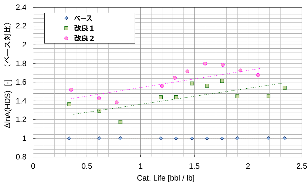
図5：積算通油量(横軸)に対する相対脱硫活性(縦軸)
