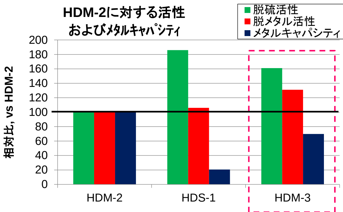
図7 市販触媒の性能比較
