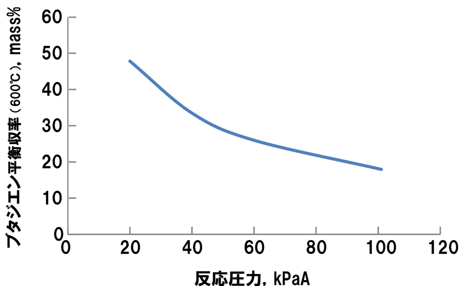
図10 圧力とブタジエン平衡収率の関係(600°C)
