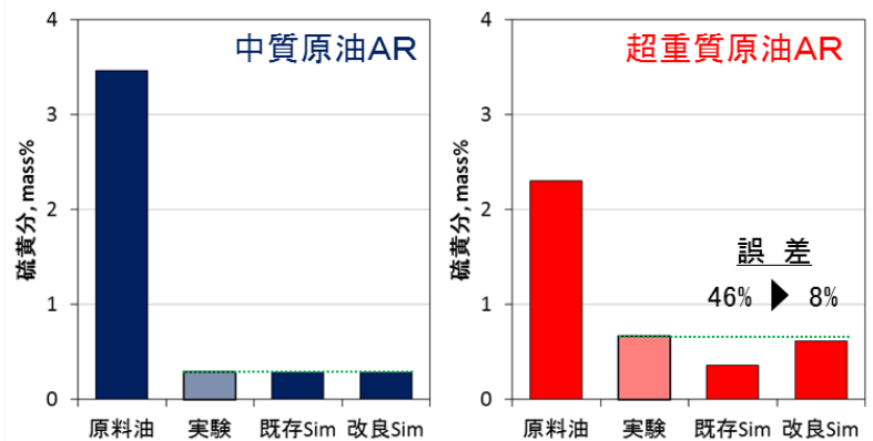
図9 RDSシミュレーションモ デルの改良結果
