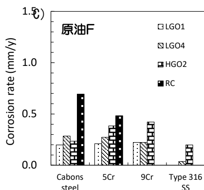
図 6.1 耐食性評価 (340°C, 原油
