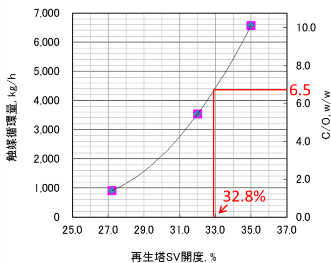
図6 再生塔SV開度と触媒循環量の関係
