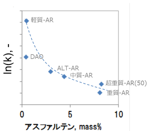
図8 RDS反応性とアスファルテンの相関 モデルの改良結果
