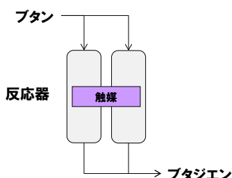
図5 ブタジエン収率向上のためのコンセプト
