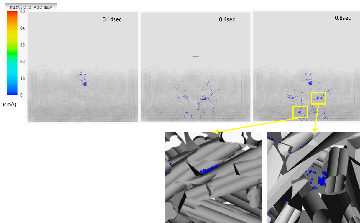
図 2：積層モデル内の粒子の滞留
