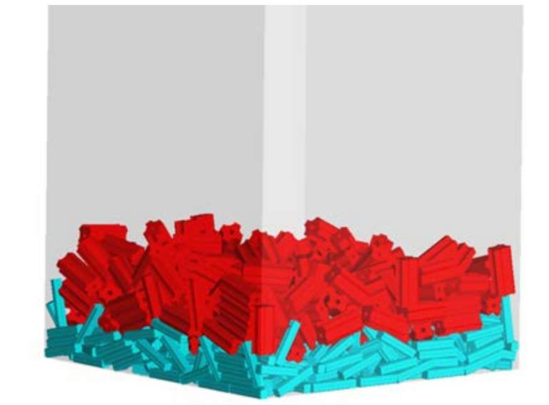
図 1 : 触媒積層のマイクロ SIM モデル
