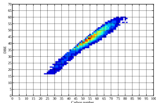
図 1 2 高セジメント VR-T の トルエン不溶-THF 可溶分の DBE プロット
