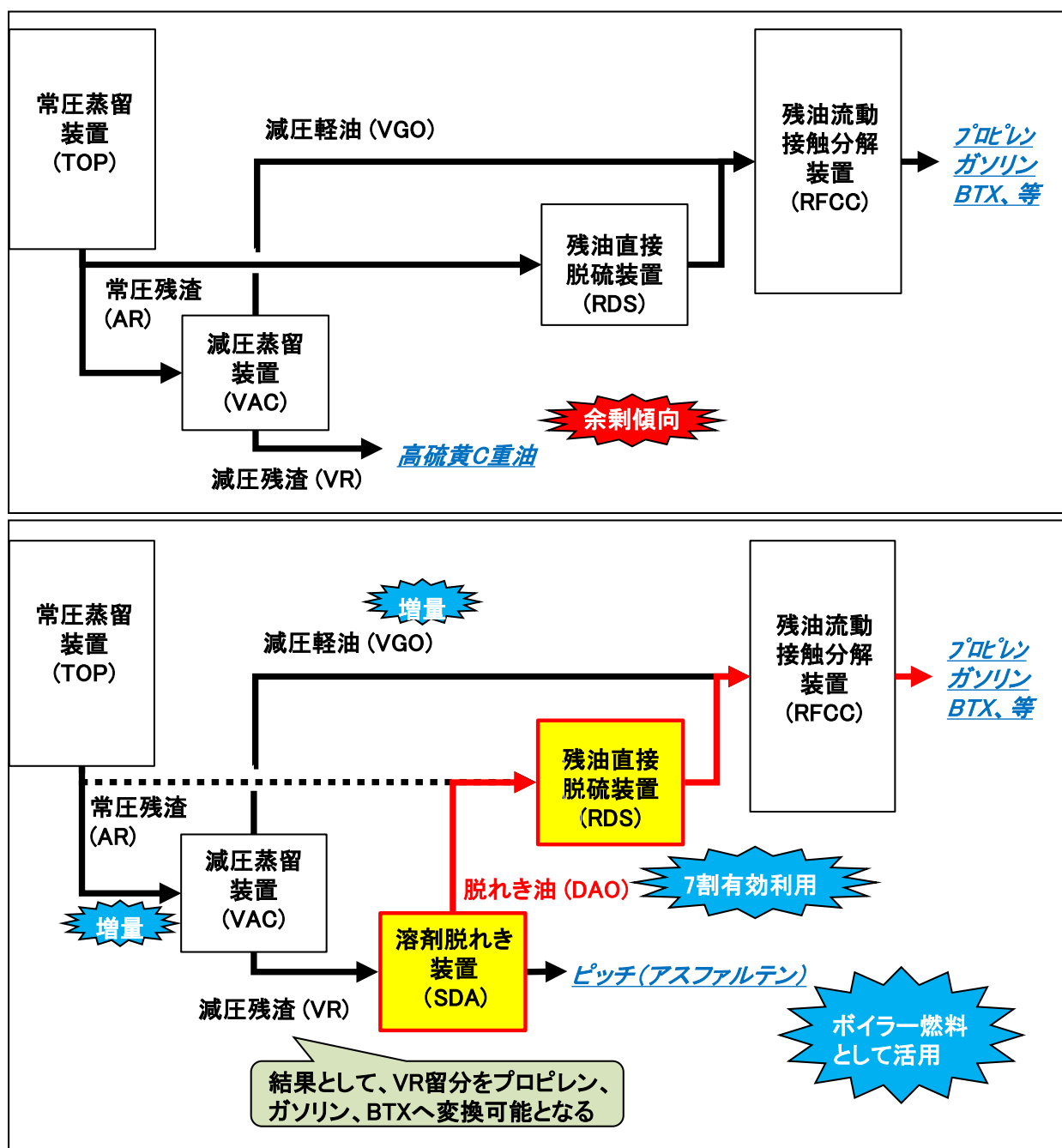
図1 従来プロセス（上）と開発プロセス（下）の比較
