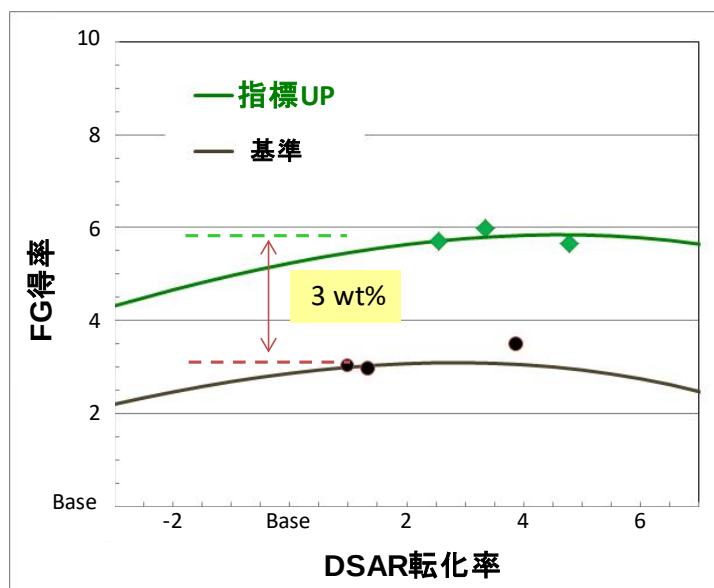
図4：RDS のシビア脱硫による指標 UP と FG 得率の向上
