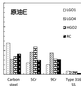
図 6.2 耐食性評価 (340°C, 原油 E)
