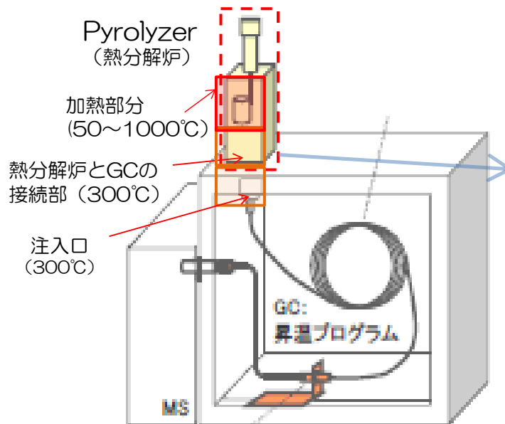
図 3.1 On-line マイクロ反応サンプラー加熱方式の熱分解ガスクロ概略図
