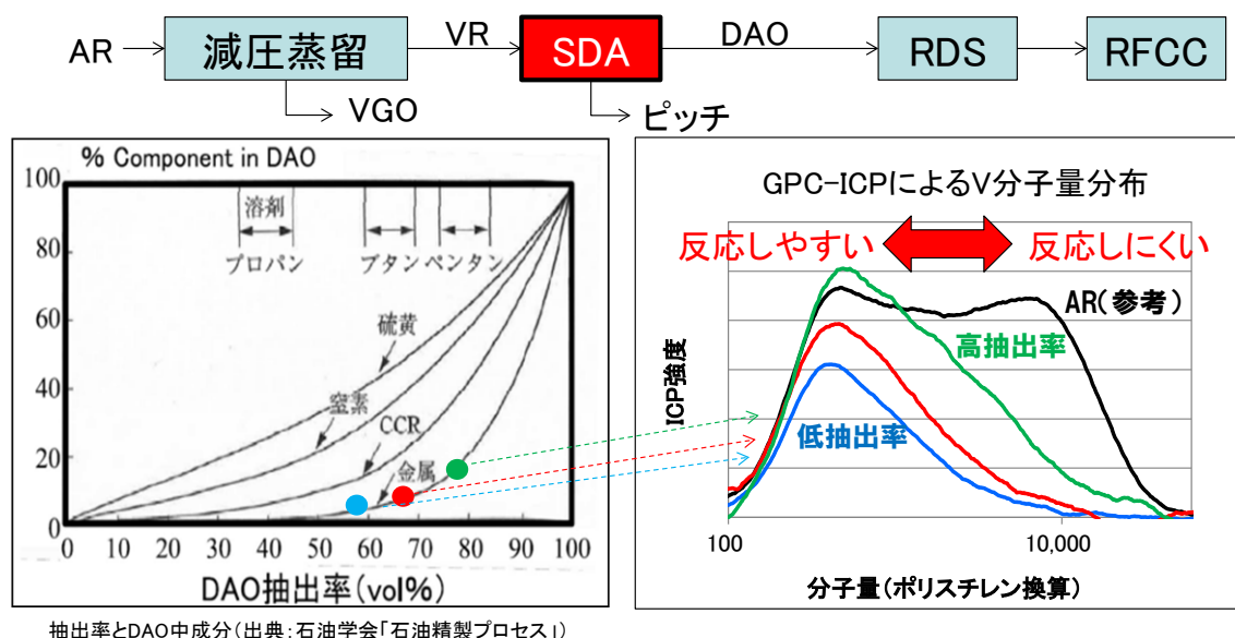
図4 抽出率が異なるDAOのGPC-ICP分析結果（バナジウム）
