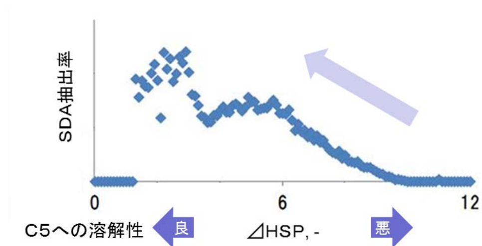
図 SDAプロセスの原料油および生成油の \Delta HSP 分布
