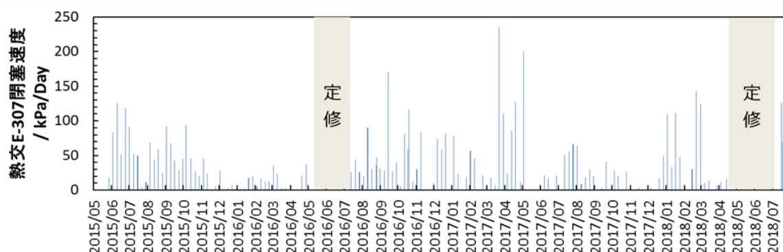
図 2 熱交閉塞速度の推移
