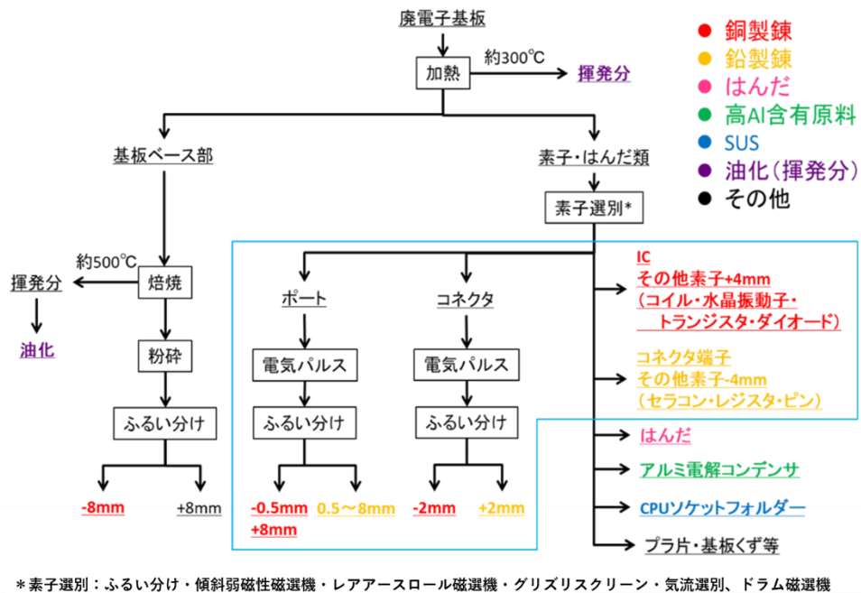
図2-4 鉛製鍊活用パターン
