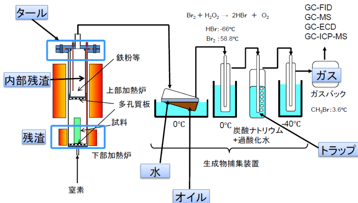
図 19 試験で使用した熱分解反応装置
