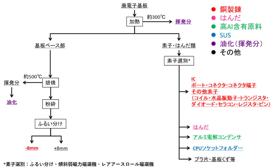
図2-3 鉛製鍊非活用パターン
