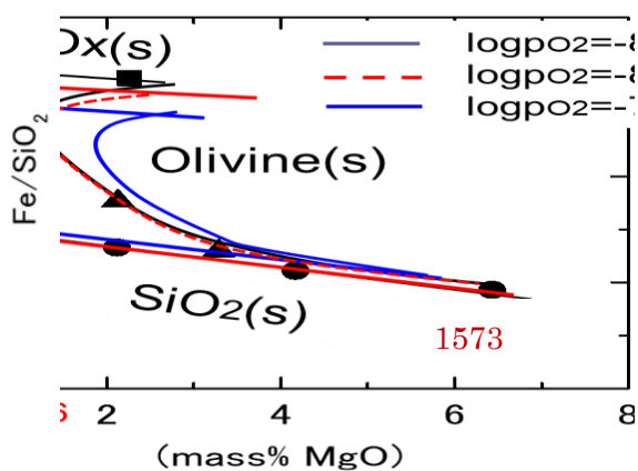
図 3 0 FeOx-SiO 2 系の液相線に及ぼす MgO 濃度と酸素分圧の影響
