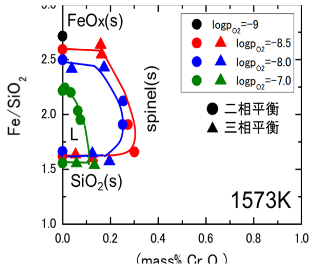
図 3 3 FeOx-SiO 2 系の液相線に及ぼす Cr 2 O 3 濃度と酸素分圧の影響
