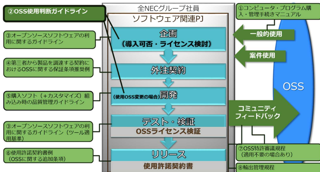
図 4.9-1 ソフトウェア関連プロジェクトの各フェーズにて参照するガイドライン群 92
