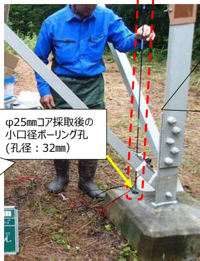
鉄塔基礎（地中部）調査方法
