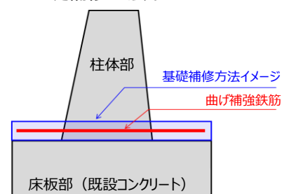
基礎補修方法イメージ
