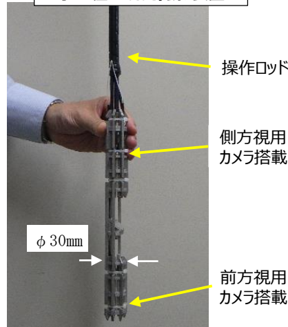
ボーリング孔に挿入する 小口径空洞内撮影装置
