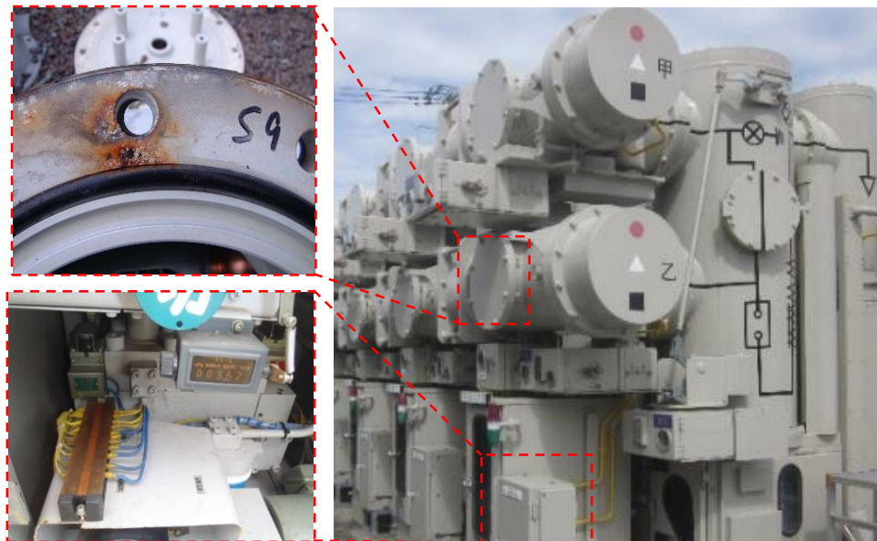
○ ローカル系GISの劣化状況
