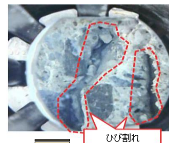
小口径空洞内撮影装置による ひび割れ個所の撮影画像
