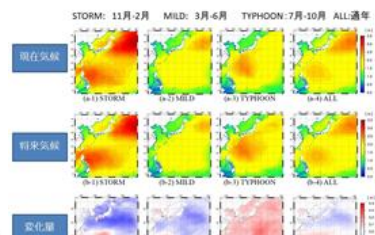
図：季節ごとの平均有最大分布の温暖化後の変化
