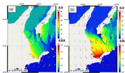
(a) 東風が吹き、根室湾の水位が上昇した。 (b) 北風に変わると、根室半島北部海域の水位が上昇した。 図：根室の高潮の説明図
