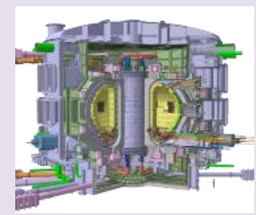
◆ 実験炉：ITER
