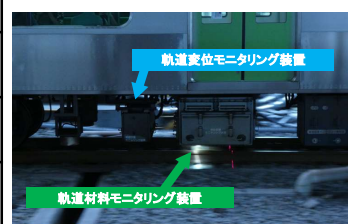
線路設備モニタリング装置
