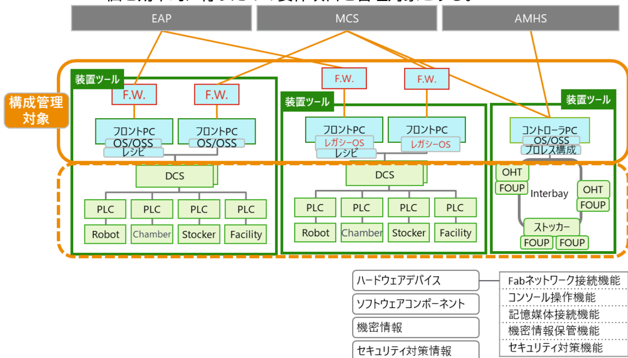
図 4-3. ファブエリアにおける構成管理対象
