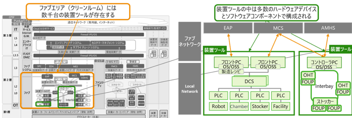
図 4-2. ファブエリアにおける資産構成
