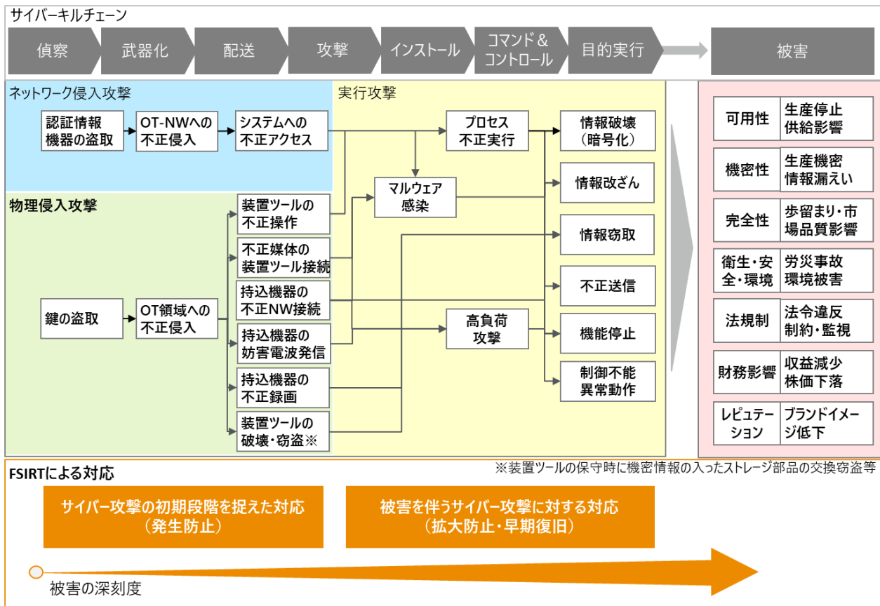
図 4-17. 工場におけるサイバーキルチェーン
