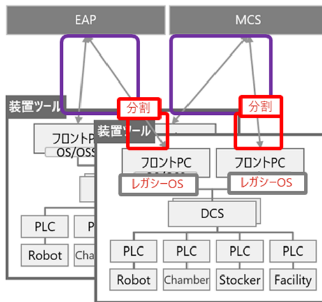
図 4-12. 装置ツールマイクロセグメンテーション構成例
