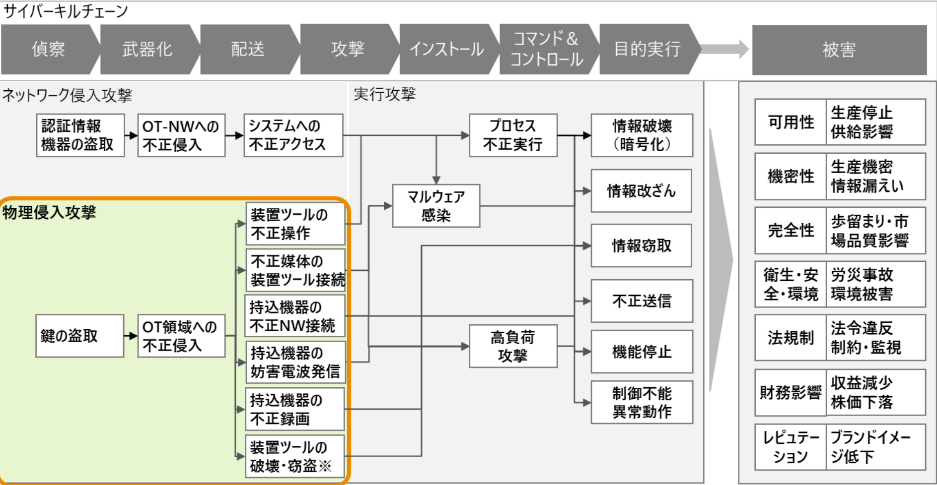
図 4-22. 工場におけるサイバーキルチェーンの物理侵入攻撃
