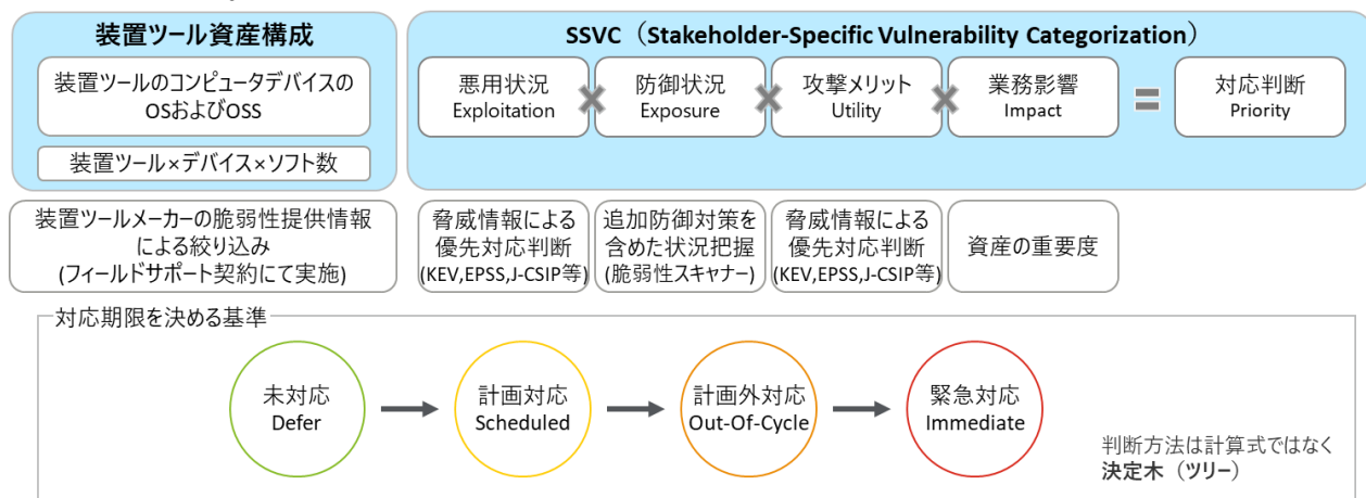
図 4-8. SSVc による脆弱性評価
