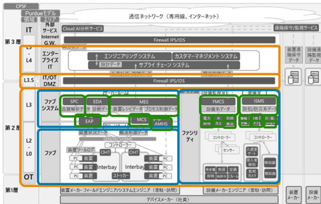
図 4-9. ネットワーク分離概要(領域・エリアレベル)
