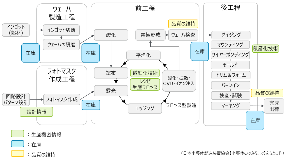
図 1-4. 半導体製造工程
