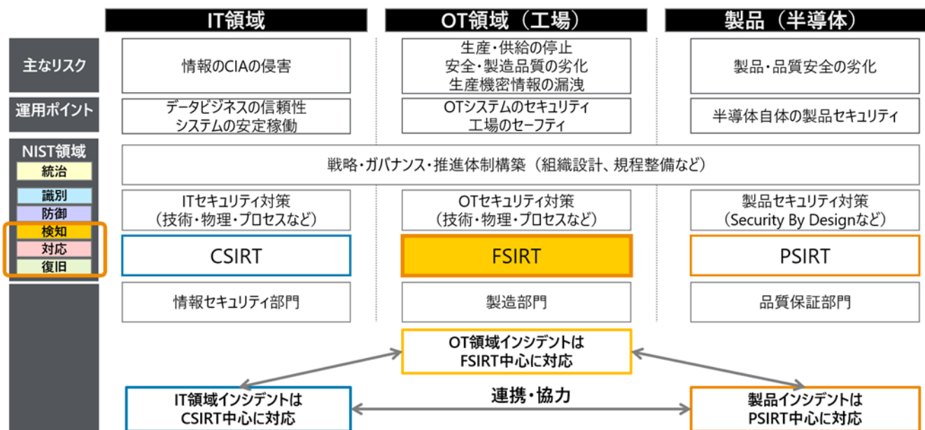
図 4-14. CSIRT、PSIRT、FSIRT の役割
