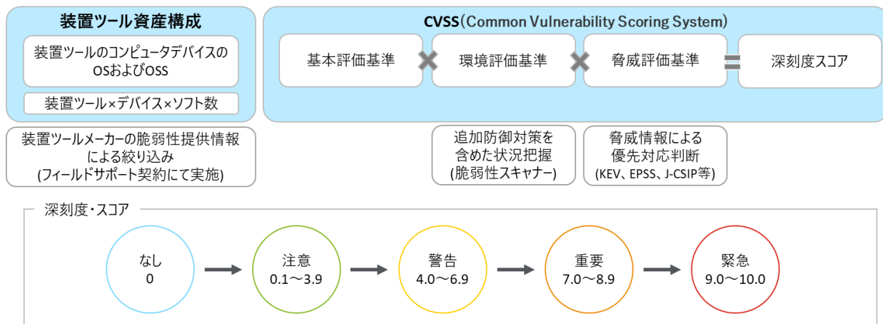
図 4-7. CVSS による脆弱性評価
