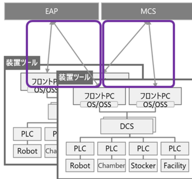
図 4-11. 装置システムネットワーク分離詳細
