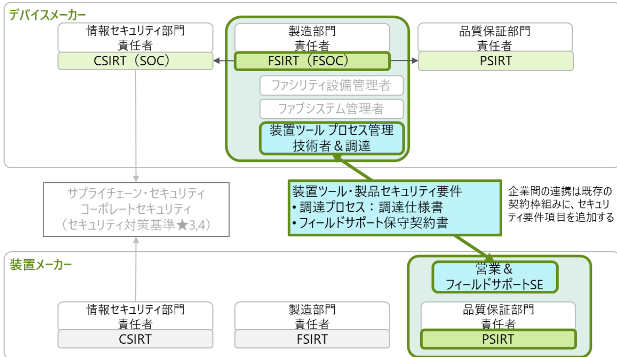
図 4-21. デバイスメーカー、装置メーカーのセキュリティ連携の具体的イメージ
