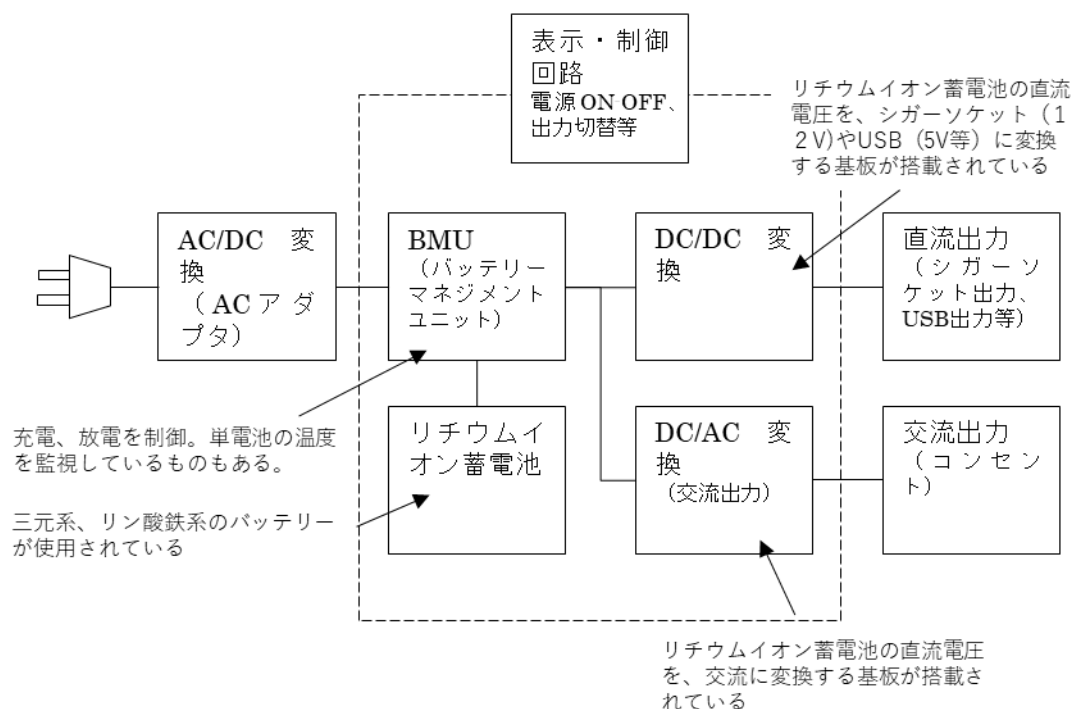
図 II-2 ポータブル電源のブロック図の例
