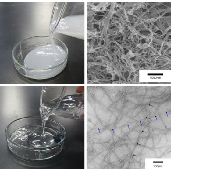
(上) 機械処理のみの従来製法によるCNF分散液 (下) TEMPO酸化法を用いた新規製法によるCNF分散液(資料提供: 日本製紙株)
