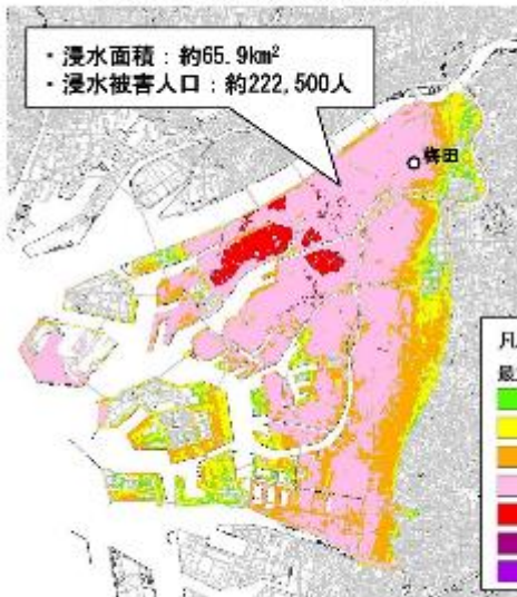
潮位によるレベル湛水による浸水状況 （高潮外力：計画高潮位0. P+5. 2m）
