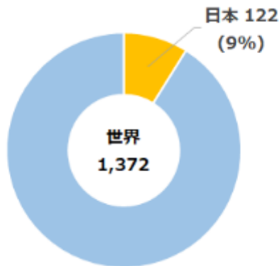
活火山数(2022年)
