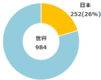
台風の数(2012～2021年)
