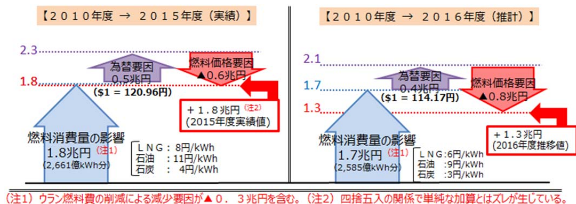
【図 1 5 原発停止に伴う燃料費増加分の要因分析】
