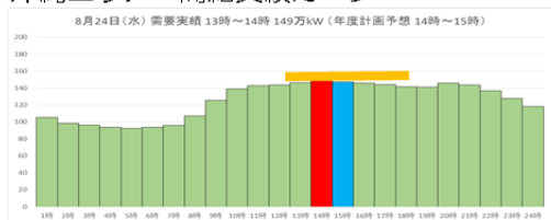
【図5 需要実績ロードカーブ(北海道、関西、九州、沖縄エリア)】
