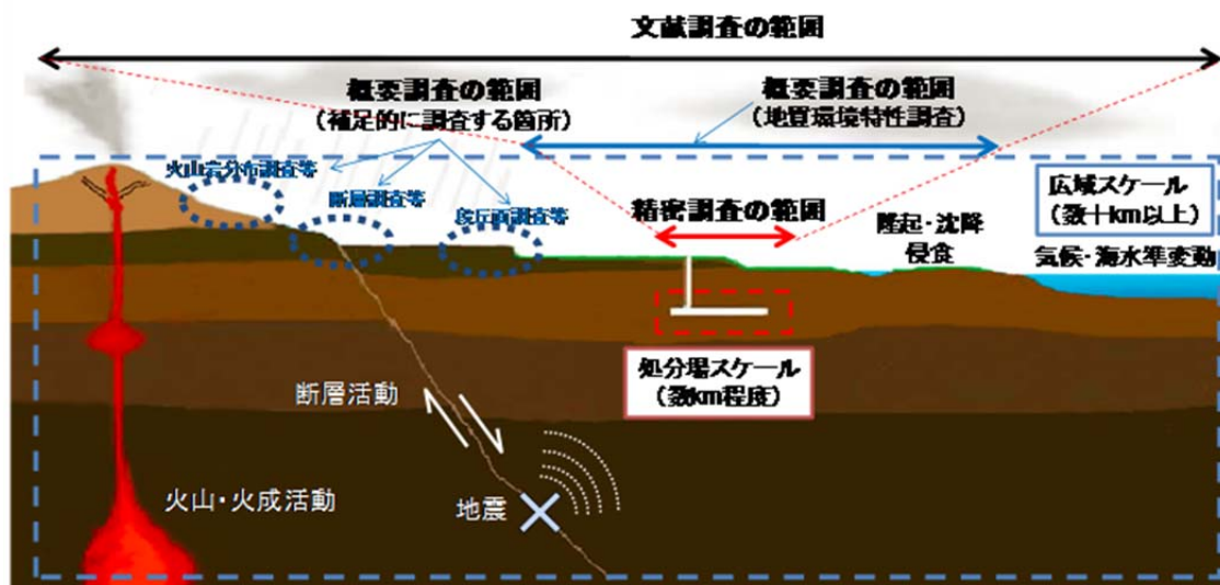
図 2 調査スケールと空間スケールの関係
