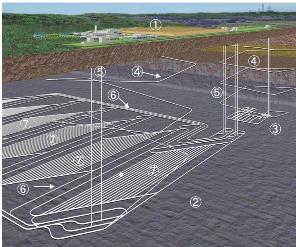
791 792 図 4.3.1.1.1 現在想定している標準的な地下施設レイアウトの例（NUMO, 2009） 793 (①地上施設、②高レベル放射性廃棄物処分場の地下施設、③地層処分低レベル放射性廃棄物処分場の地 794 下施設、④斜坑、⑤立坑、⑥連絡坑道、⑦処分パネル（処分坑道の集合した区画）)
