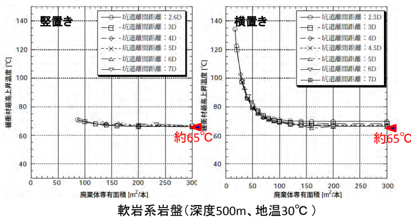
図 3.3.1.2 廃棄体の暖め合う効果を見捨てるほど距離を離れた場合の緩衝材最高上昇温度（第 2 次取りまとめ(JNC, 1999c)に加筆）
