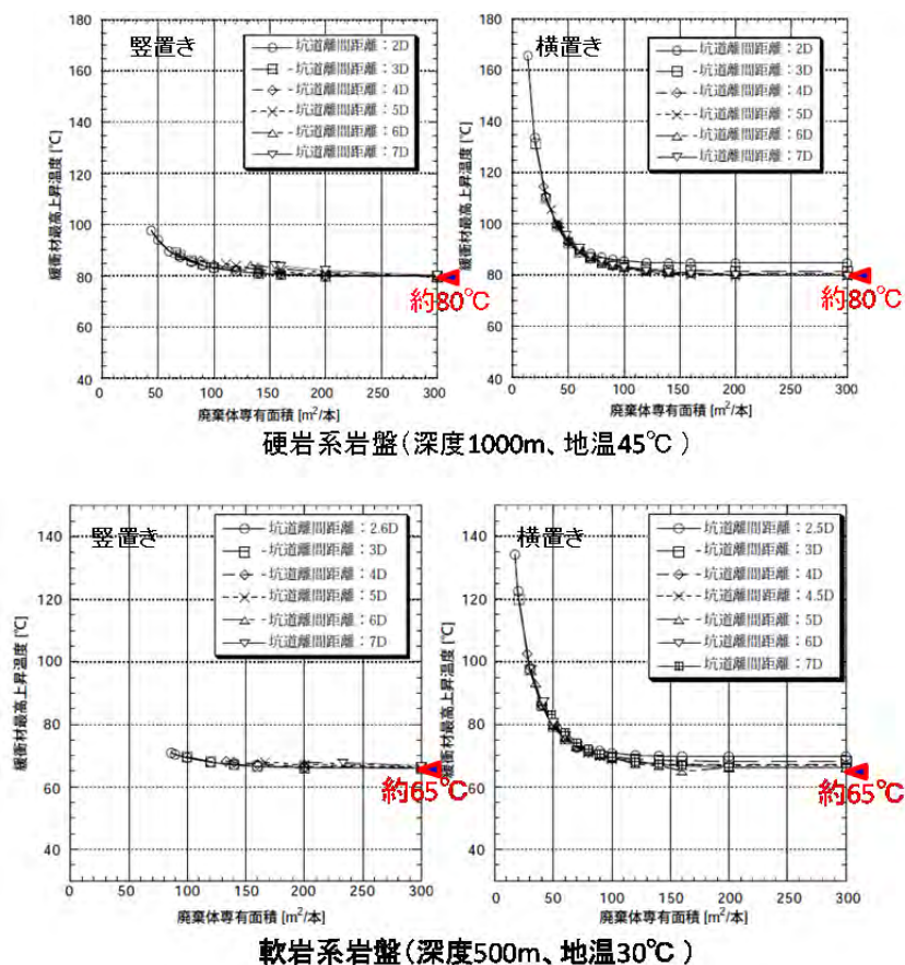
図 3.3.1.2 廃棄体の暖め合う効果を見捨てるほど距離を離れた場合の緩衝材最高上昇温度 (第 2 次取りまとめ(JNC, 1999c)に加筆)
