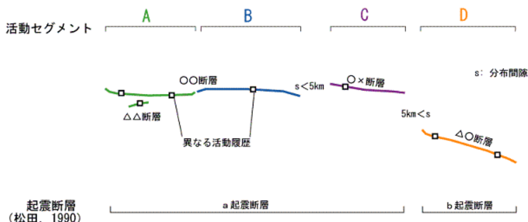
図 3.3.1.4 活動セグメントと起震断層の模式図（産業技術総合研究所ウェブサイト）
