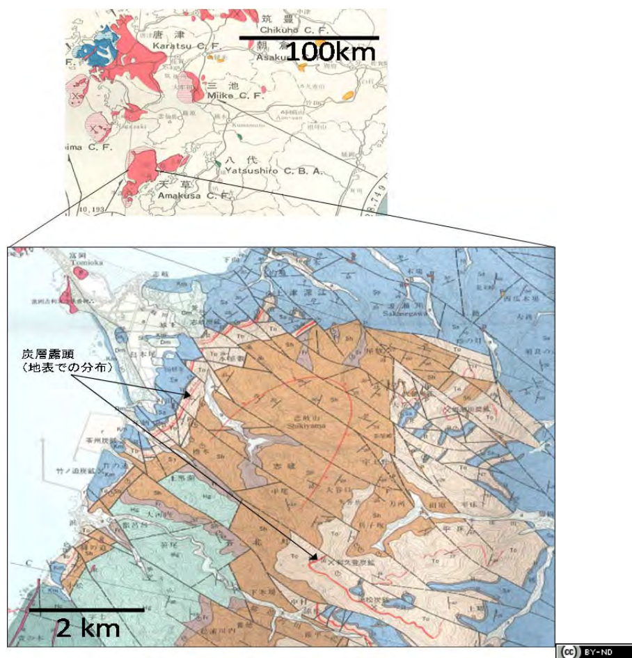
図 3.3.1.7 「日本炭田図（第2版）」（産業技術総合研究所，1973）と個別地点（天草炭田図（5万分の1）（産業技術総合研究所，1997））における図の例 44
