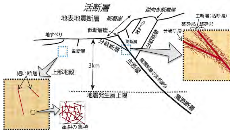
断層活動が及ぼす影響 (山崎 (2013) 第 2 図に加筆)
