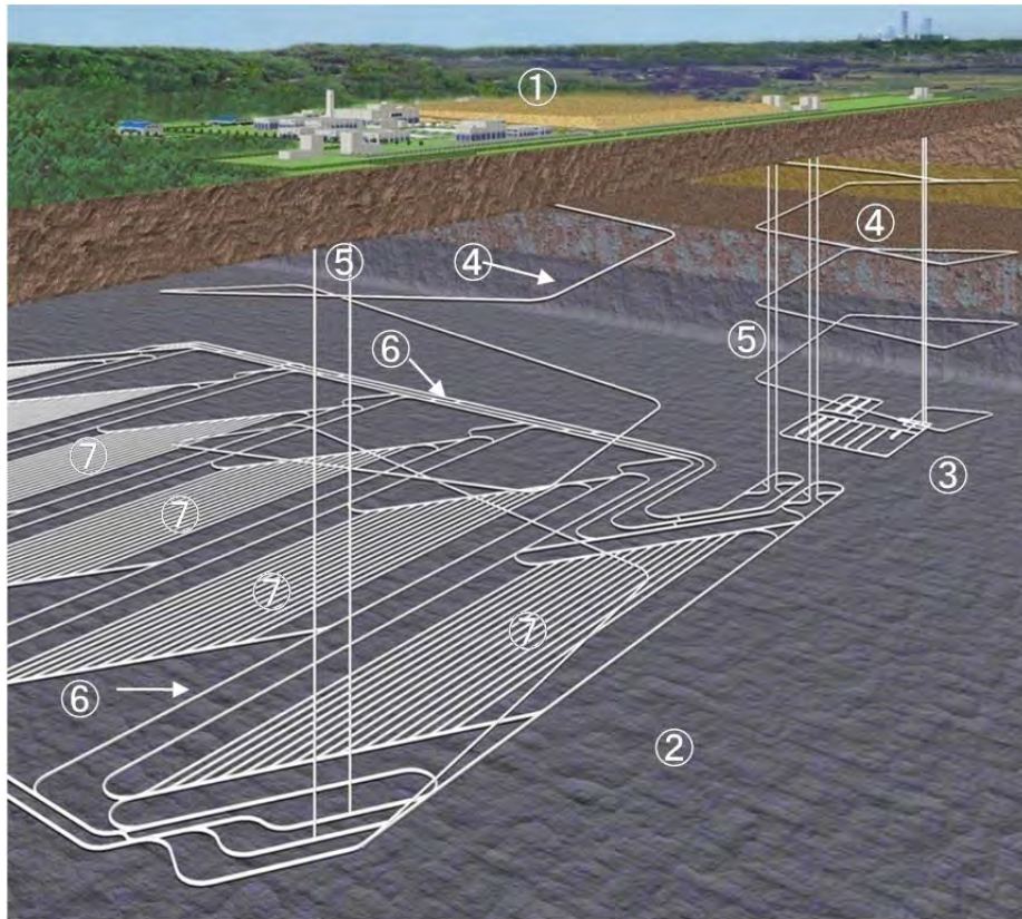
図 3.4.1 NUMOが想定している標準的な地下施設レイアウトの例（NUMO, 2009b）
