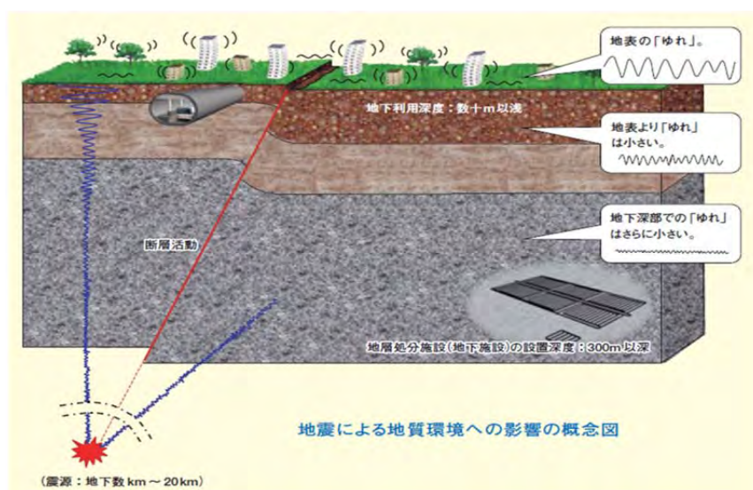
図 3.3.1.5 地震による地質環境への影響の概念図（(NUMO, 2009a) を一部修正）
