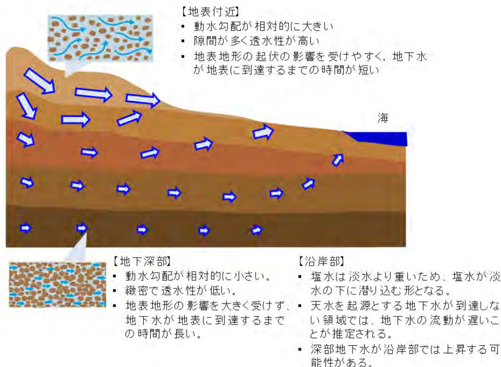
図 3.3.1.6 地表付近と地下深部における地下水の流れ（模式図）
