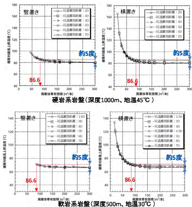
図 3.3.1.3 廃棄体専有面積 86.6m 2 の場合の緩衝材最高上昇温度 (第2次取りまとめ(JNC, 1999c)に加筆)
