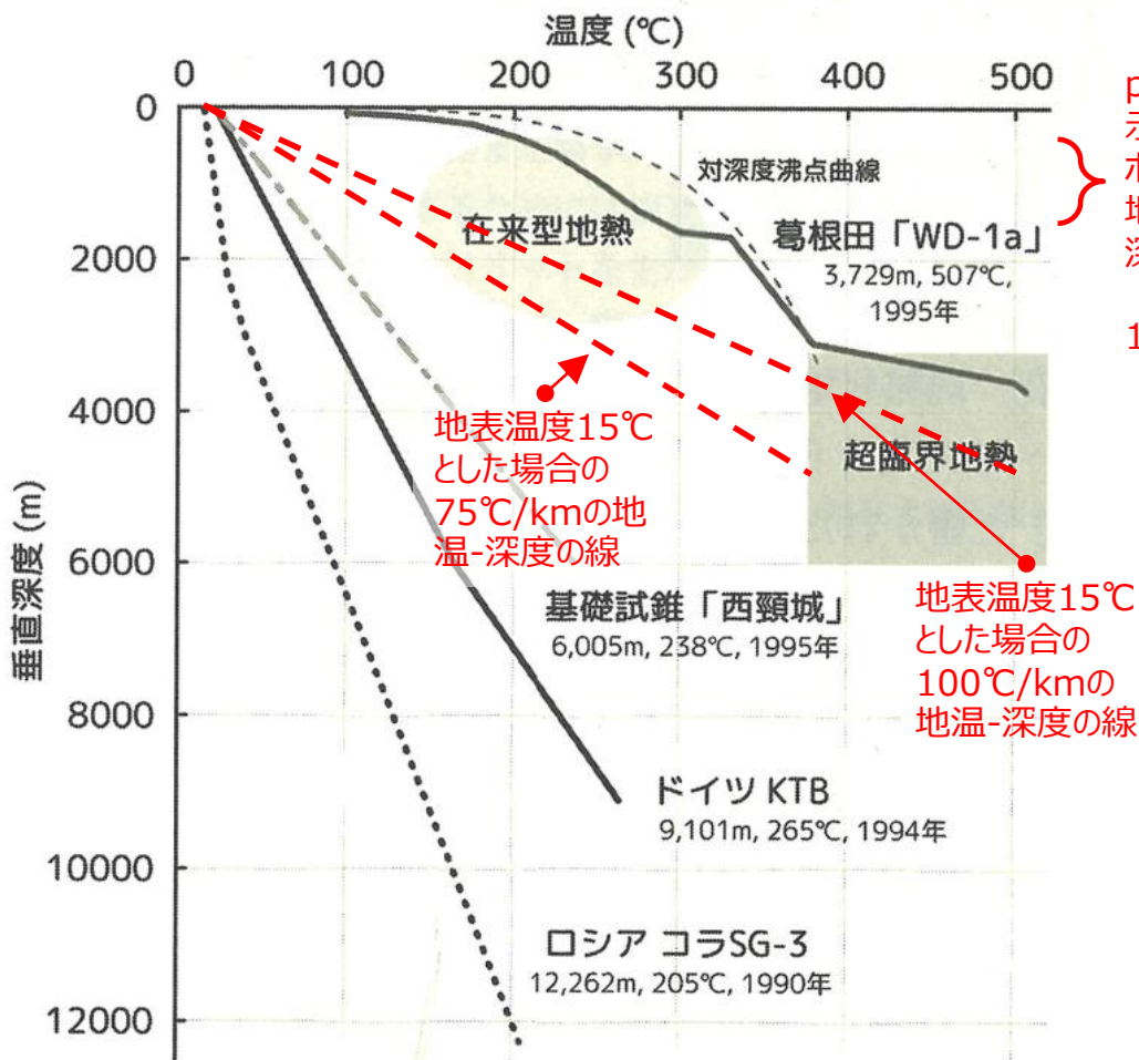
図 17-1 代表的な大深度及び高温掘削の深度と地層温度
