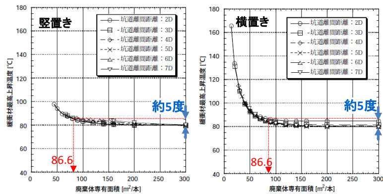
硬岩系岩盤(深度1000m、地温45°C)
