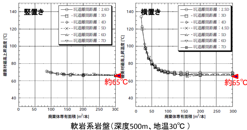
図 3.3.1.2 廃棄体の暖め合う効果が無視できるほど距離を離れた場合の緩衝材最高地上昇温度（第 2 次取りまとめ(JNC, 1999c)に加筆）
