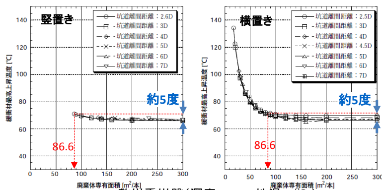
軟岩系岩盤(深度500m、地温30°C)
