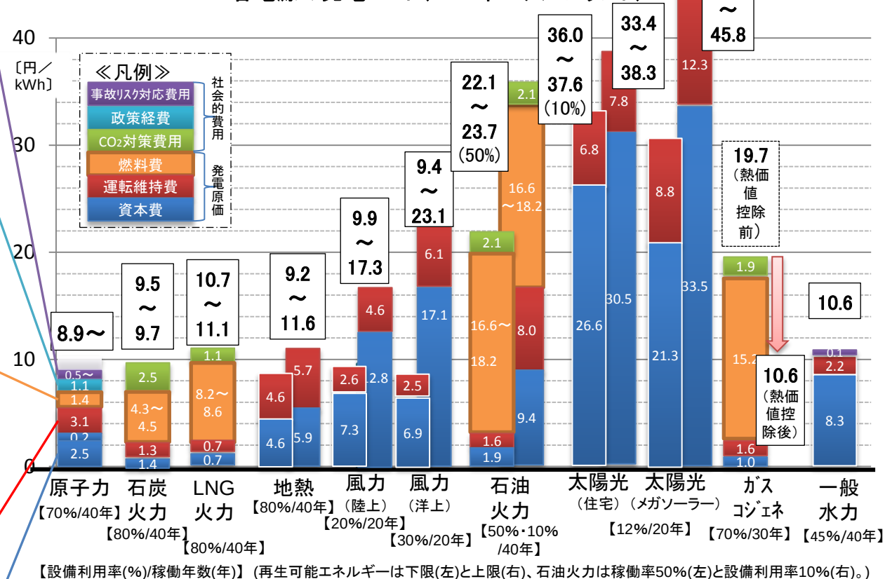
各電源の発電コスト(2010年モデルプラント)
