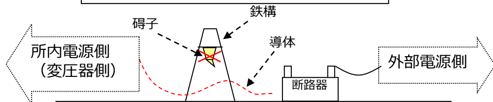
1 相開放故障の概要
