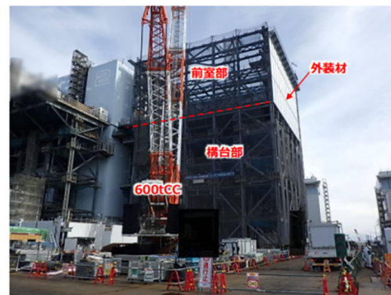
2号機南側構台設置の状況
