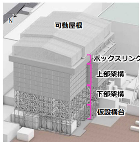
1号機大型カバー概要図
