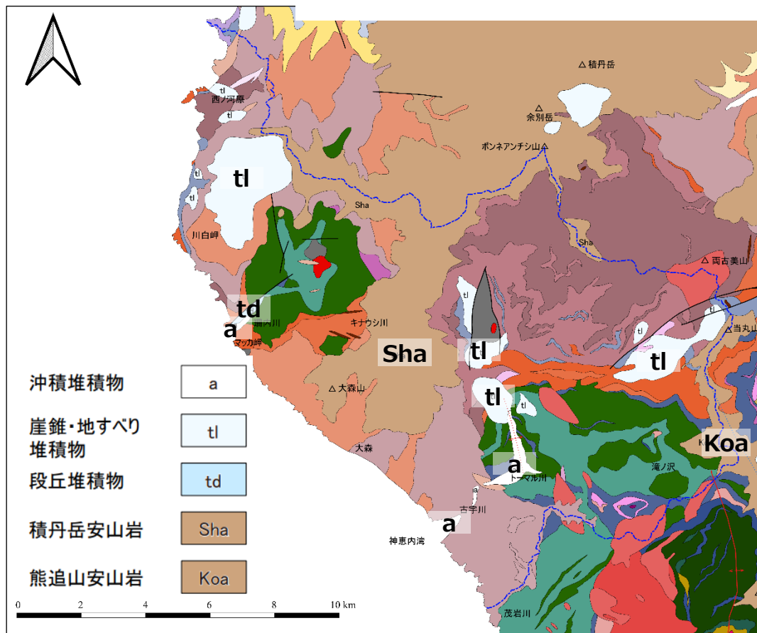
文献調査対象地区および周辺陸域地質図
