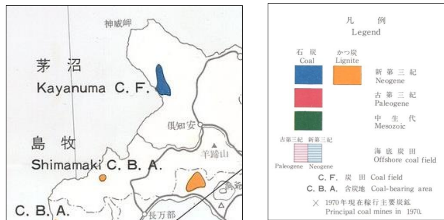
日本炭田図（徳永他，1973）より抜粋し加筆
