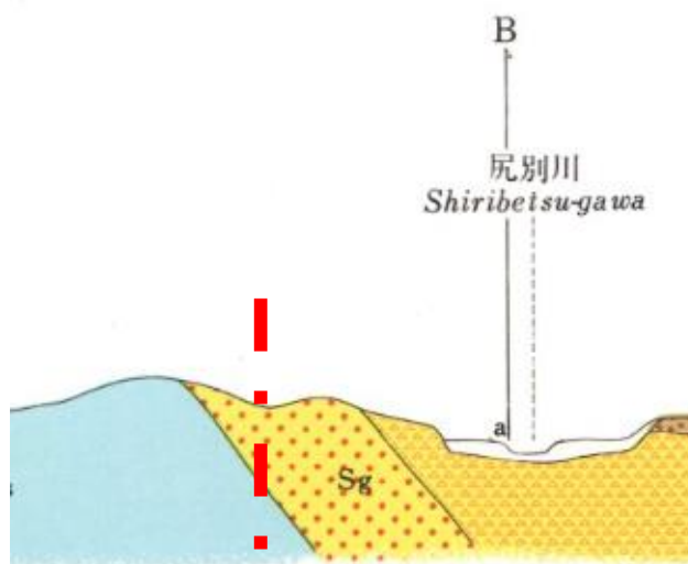
山岸ほか（1976）における尻別川層(瀬棚層)の分布状況
