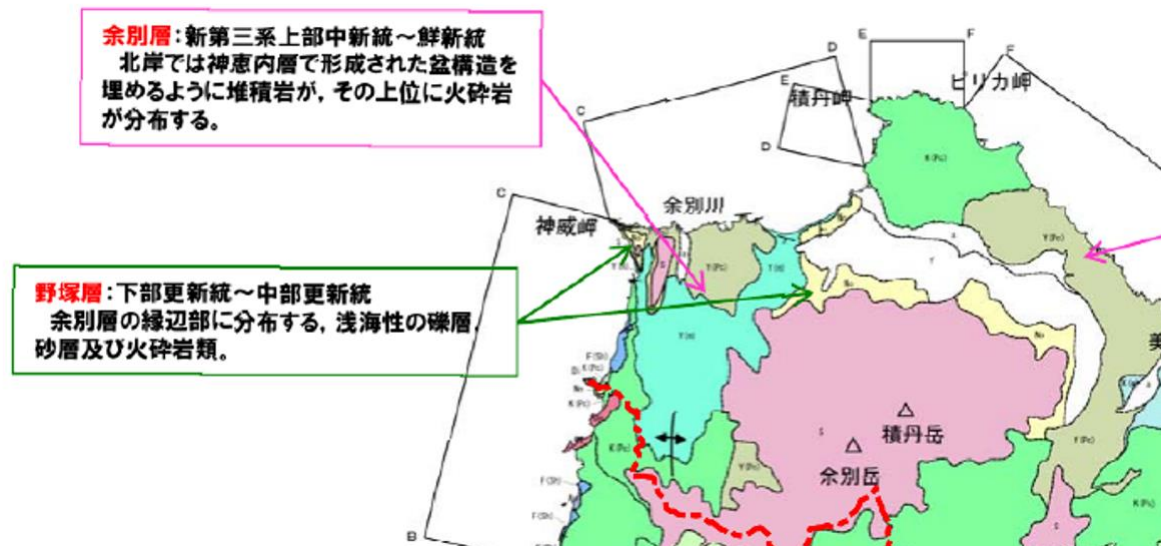
北海道電力（2016b）における野塚層の分布状況 北海道電力（2016b）に神恵内村の行政界を赤点線で加筆。
