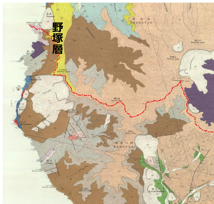
山岸・石井（1979）における野塚層の分布状況 山岸・石井（1979）に神威内村の市町村境界を赤点線で加筆。
