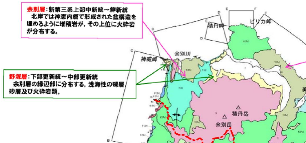
北海道電力（2016b）における野塚層の分布状況 北海道電力（2016b）に神威内村の行政界を赤点線で加筆。
